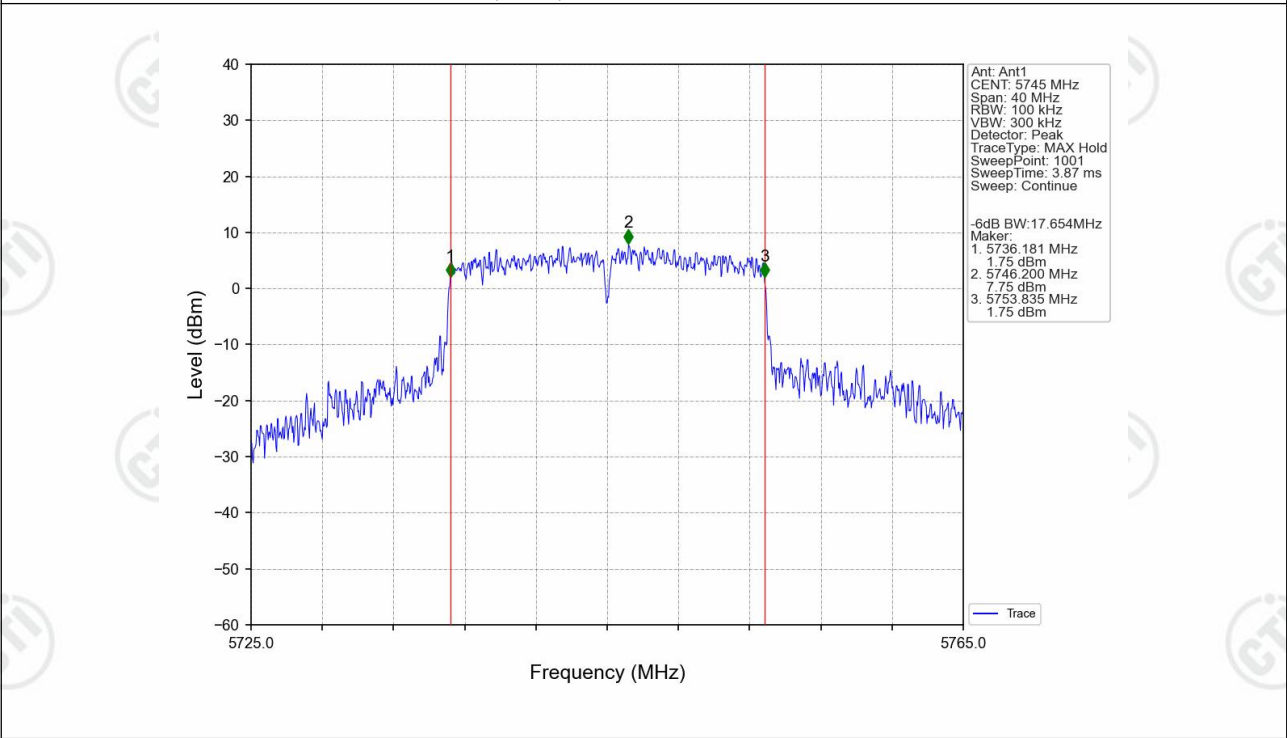
802.11n(HT20)_LCH_5745MHz_Ant1_NTNV
