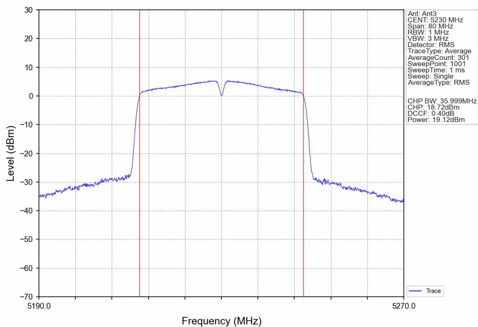
802.11n(HT40)_HCH_5230MHz_Ant3_NTNV
