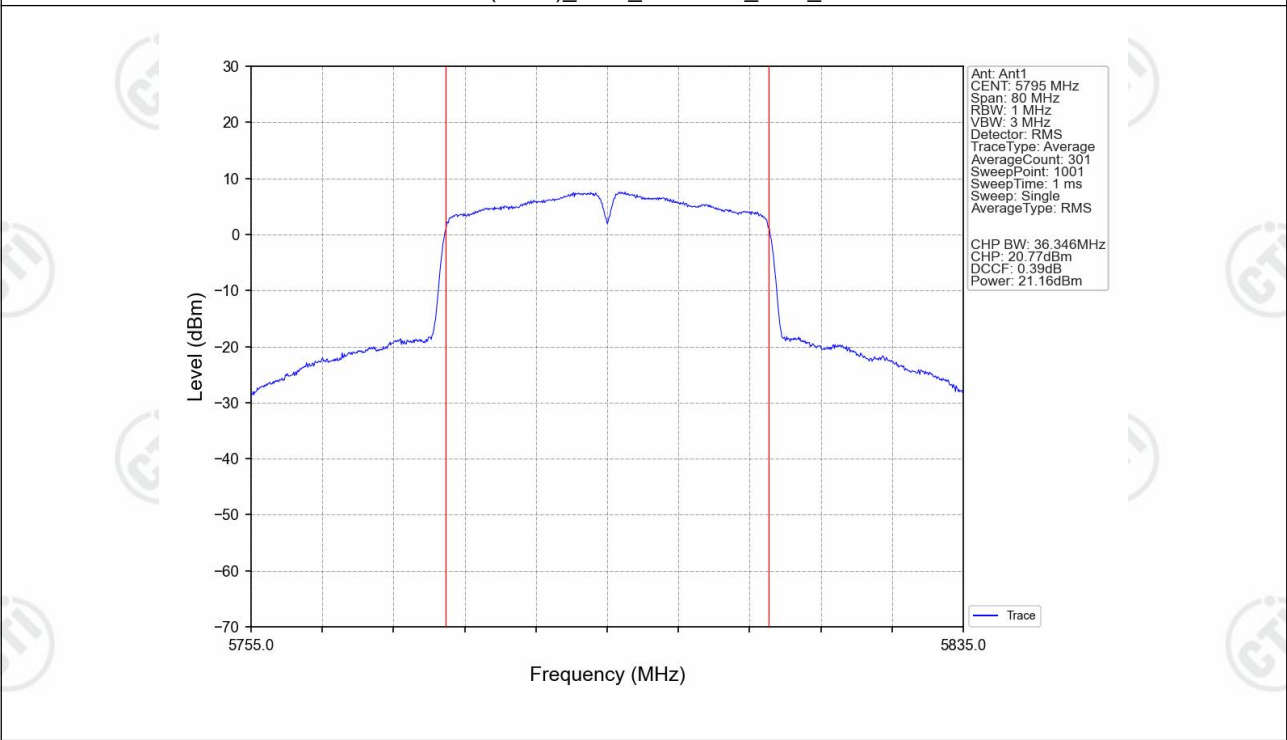
802.11n(HT40)_HCH_5795MHz_Ant1_NTNV
