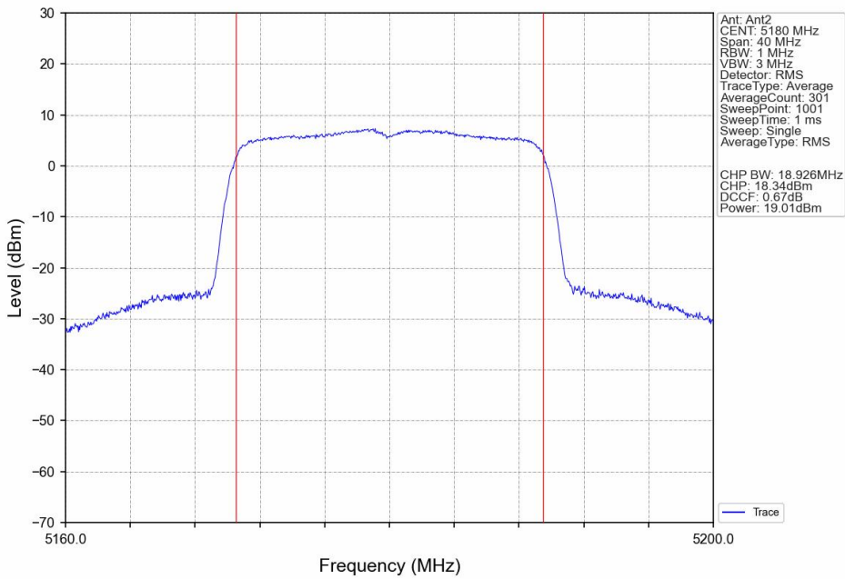
802.11be(EHT20)_LCH_5180MHz_SU_ / _Ant2_NTNV
