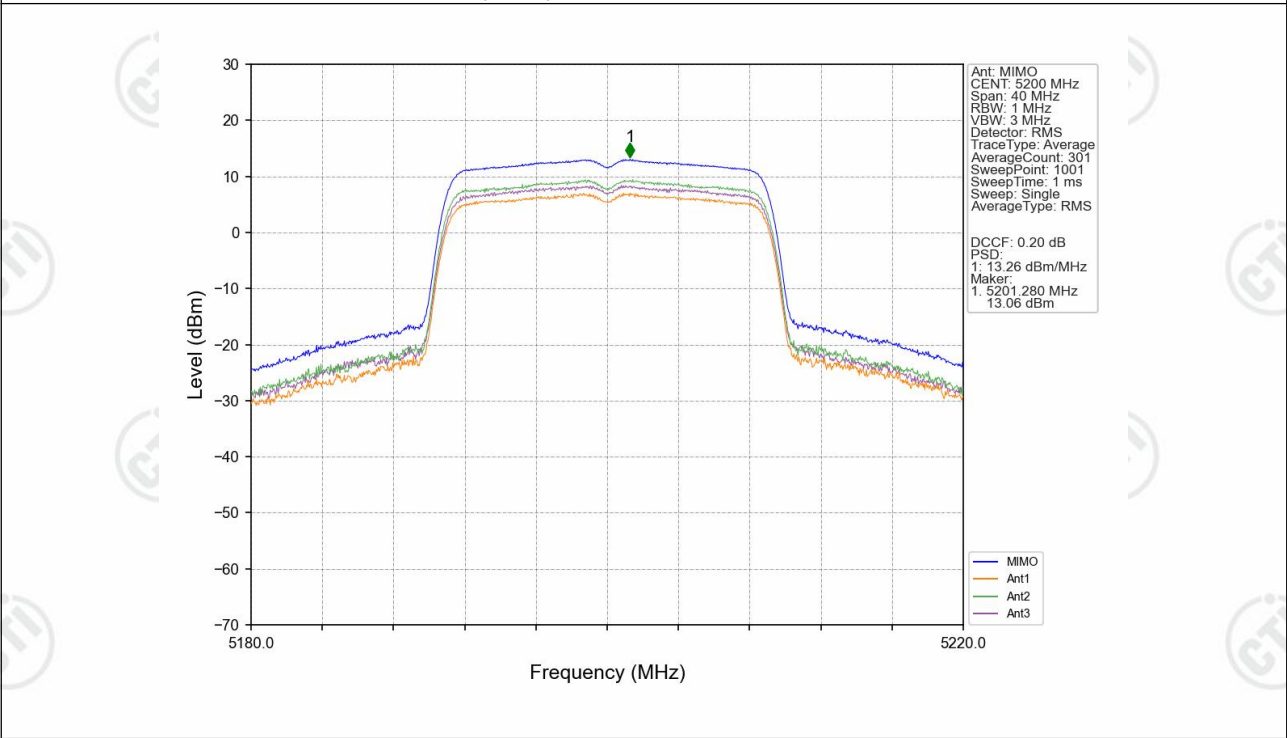
802.11n(HT20)_MCH_5200MHz_MIMO_NTNV
