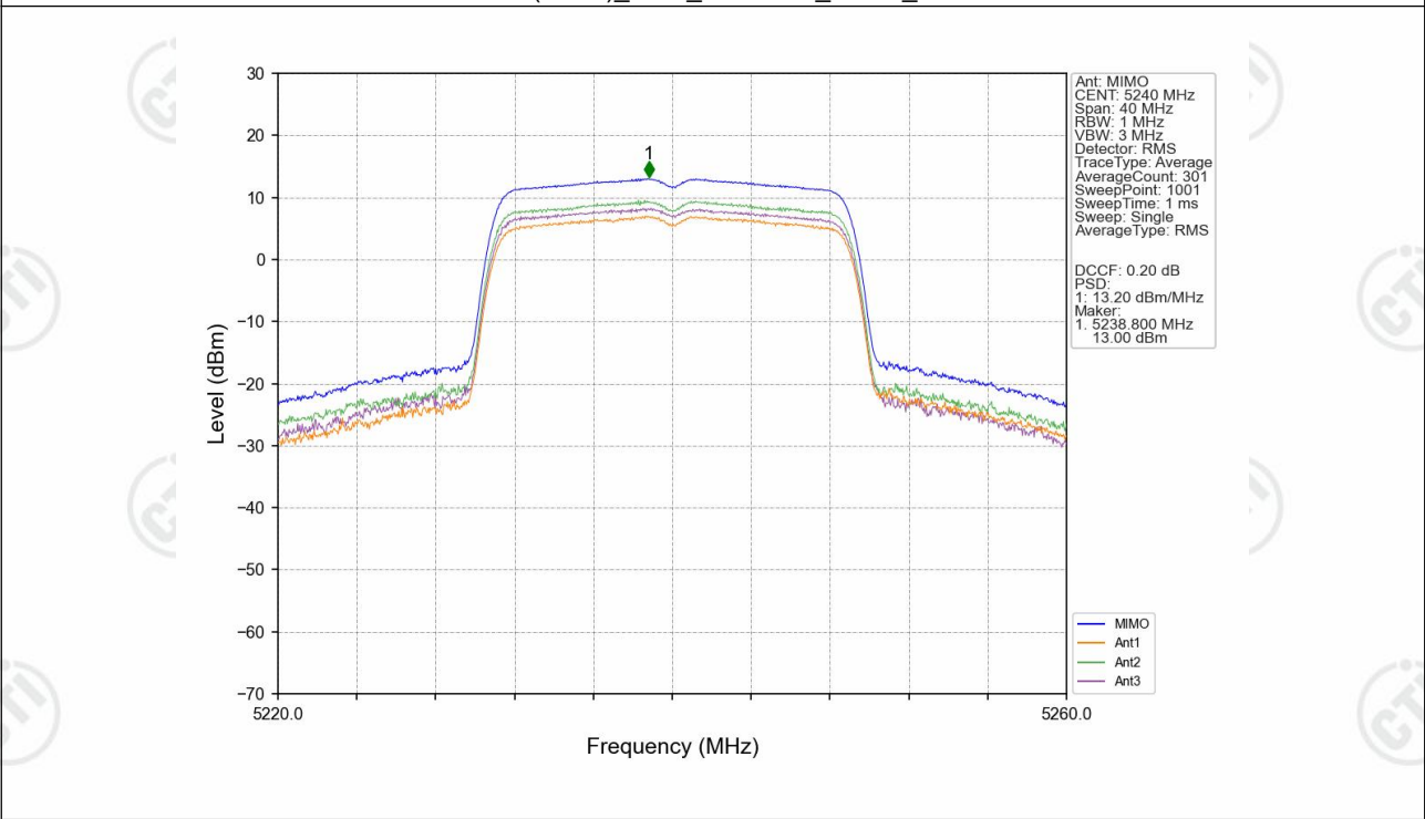
802.11n(HT20)_HCH_5240MHz_MIMO_NTNV
