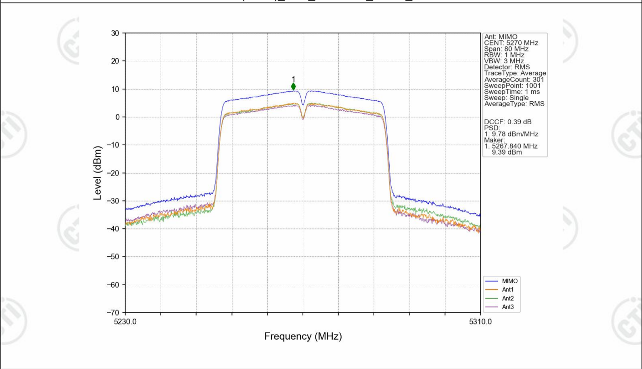
802.11n(HT40)_LCH_5270MHz_MIMO_NTNV
