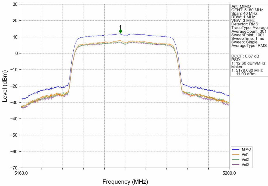
802.11be(EHT20)_LCH_5180MHz_SU_ / _MIMO_NTNV
