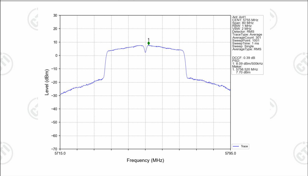
802.11n(HT40)_LCH_5755MHz_Ant1_NTNV
