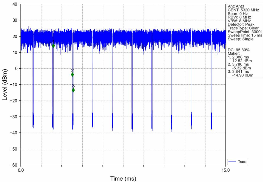
802.11a_HCH_5320MHz_Ant3_NTNV
