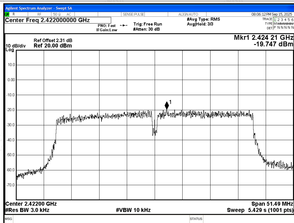
PSD NVNT be40 2422MHz Ant2
