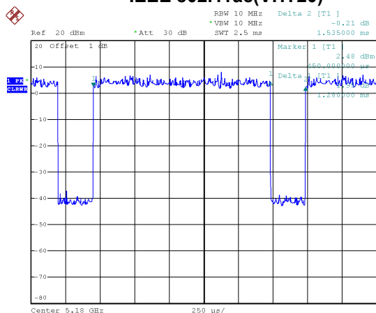
IEEE 802.11ac(VHT20)
