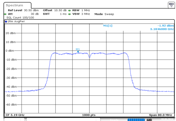
n40_5190MHz_Chain 1
