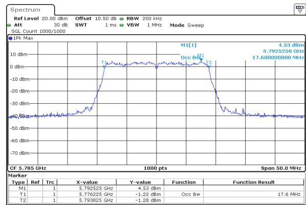
ac20_5785MHz_Chain 0
