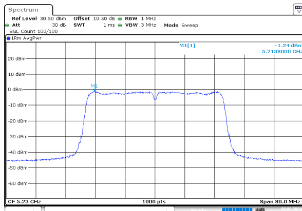
n40_5230MHz_Chain 0
