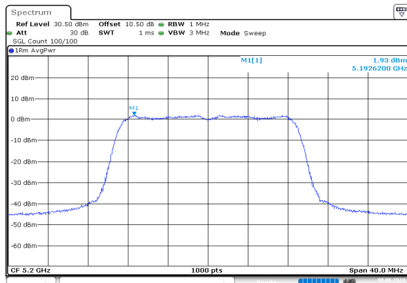
ac20_5200MHz_Chain 0
