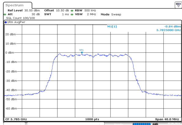
ac20_5785MHz_Chain 1
