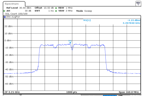
ac80_5210MHz_Chain 1
