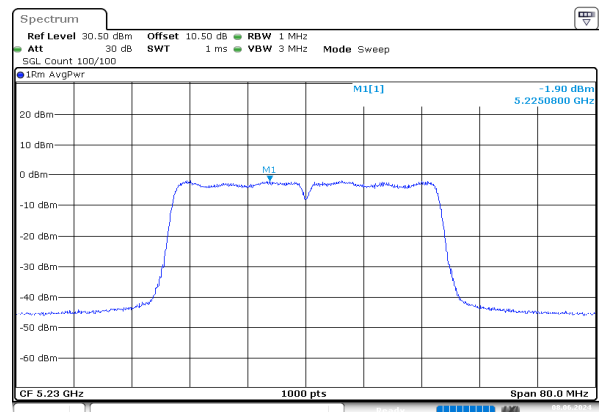
n40_5230MHz_Chain 1
