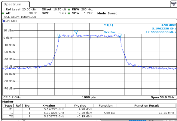
ac20_5200MHz_Chain 0
