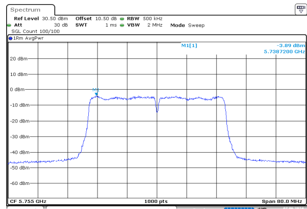
n40_5755MHz_Chain 1
