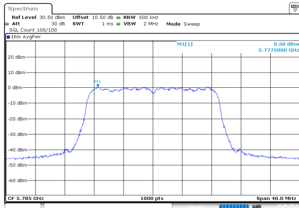
ac20_5785MHz_Chain 0
