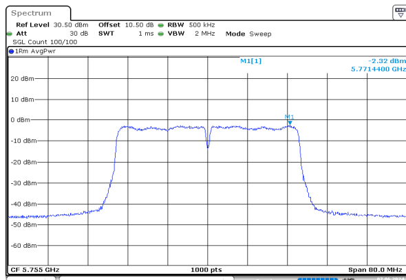
n40_5755MHz_Chain 0
