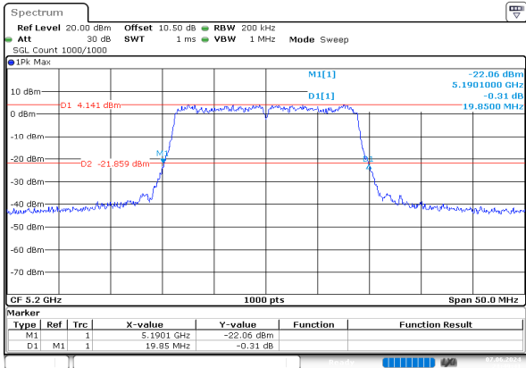
ac20_5200MHz_Chain 0
