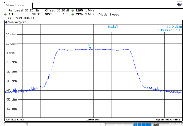
a_5200MHz_Chain 1
