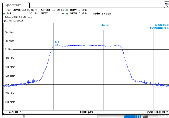
a_5200MHz_Chain 0
