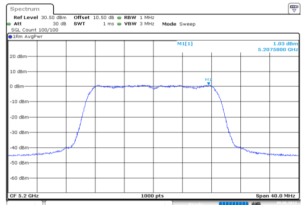
ac20_5200MHz_Chain 1
