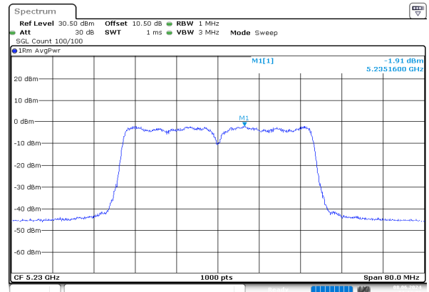
ac40_5230MHz_Chain 1
