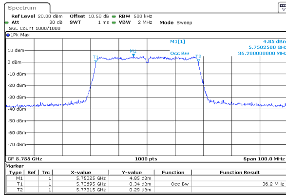
n40_5755MHz_Chain 0
