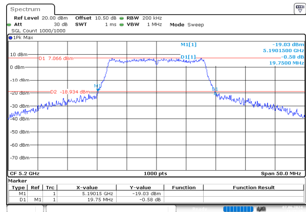
a_5200MHz_Chain 0
