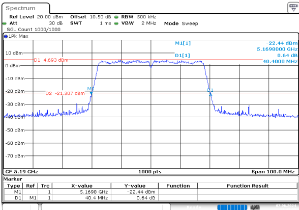
n40_5190MHz_Chain 0
