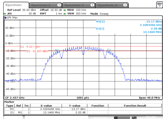
b_2437MHz_Chain 0
