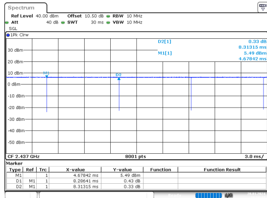
b_2437MHz_Chain 0
