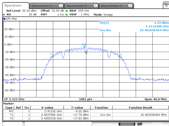
b_2412MHz_Chain 0
