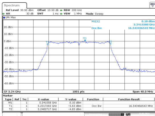
a_ 5240MHz_Chain 0
