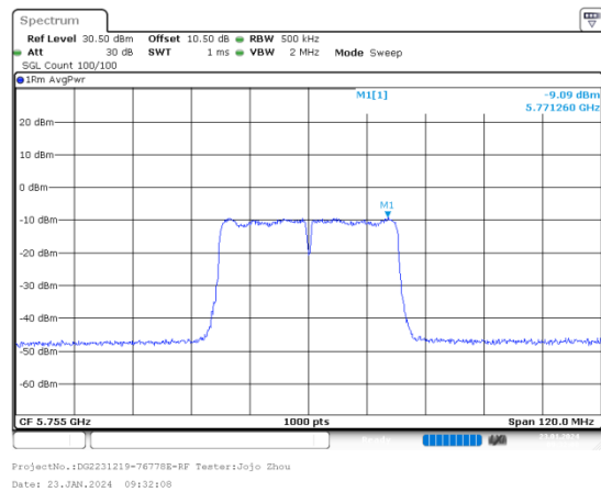
n40_5755MHz_Chain 0
