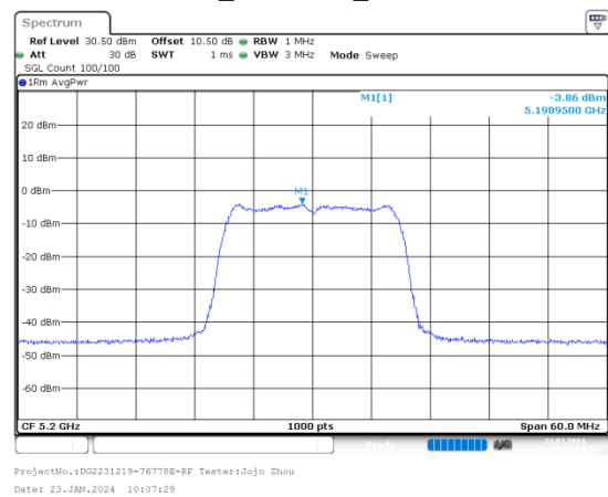
ac20_5200MHz_Chain 1
