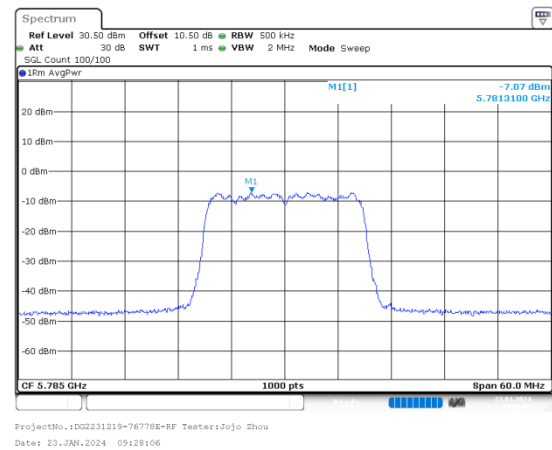
ac20_5785MHz_Chain 0
