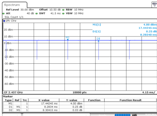
b_2437MHz_Chain 0
