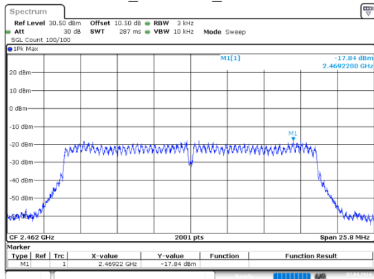
n20_2462MHz_Chain 0
