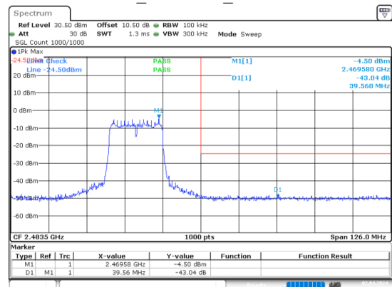
n20_2462MHz_Chain 0
