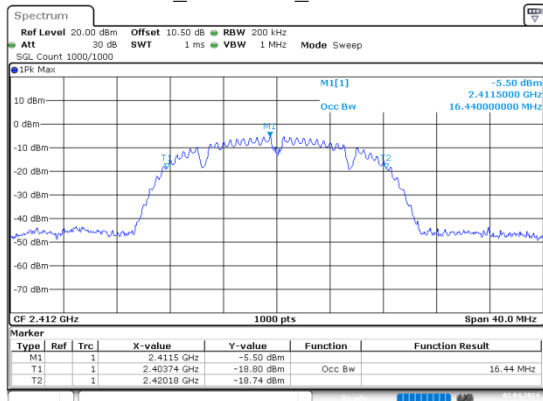
b_2412MHz_Chain 0
