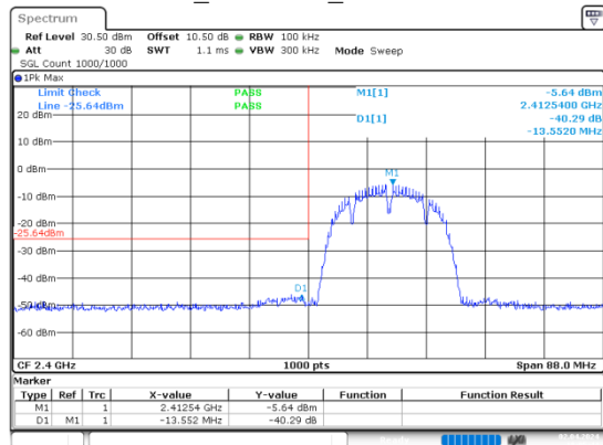
b_2412MHz_Chain 0
