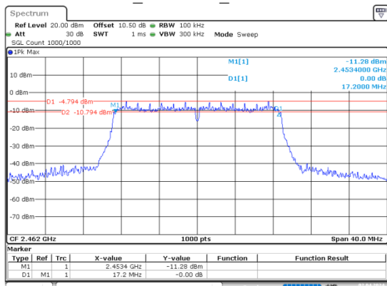
n20_2462MHz_Chain 0
