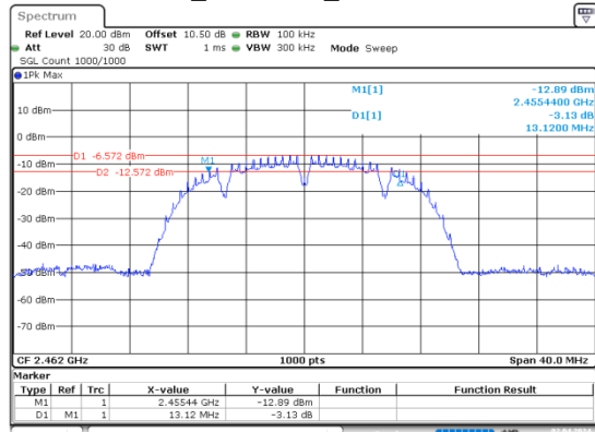
b_2462MHz_Chain 0
