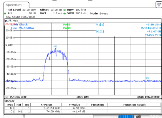
b_2462MHz_Chain 0
