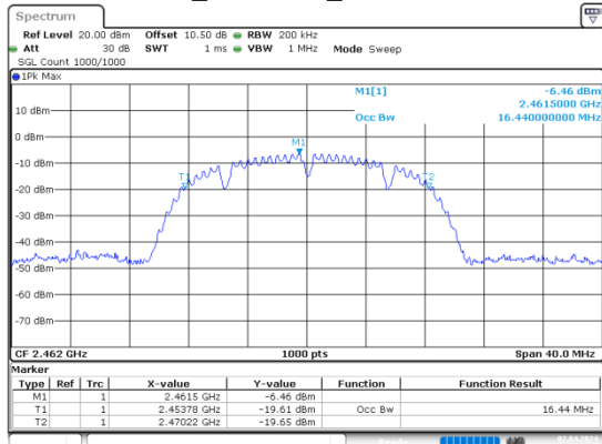
b_2462MHz_Chain 0
