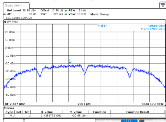
b_2437MHz_Chain 0
