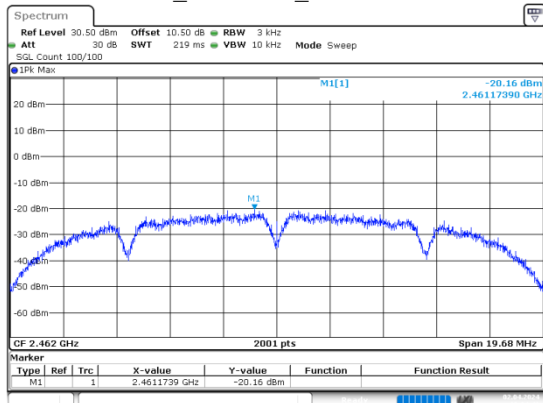
b_2462MHz_Chain 0
