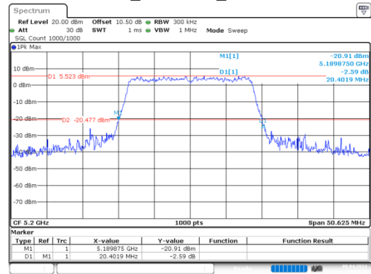
ac20_5200MHz_Chain 0
