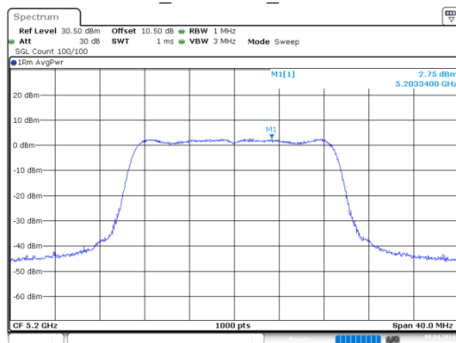
ac20_5200MHz_Chain 0
