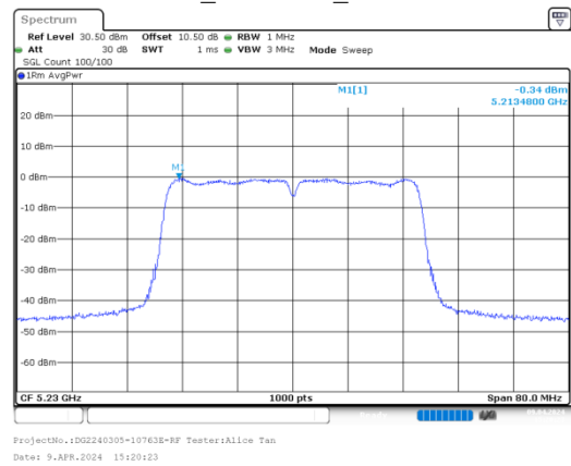
ac40_5230MHz_Chain 1
