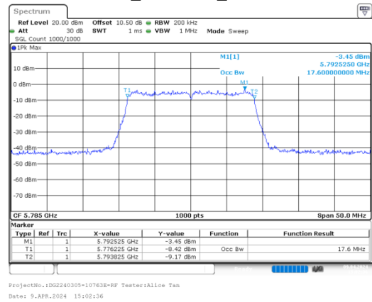
ac20_5785MHz_Chain 0
