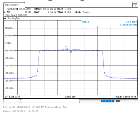
ac80_5210MHz_Chain 1
