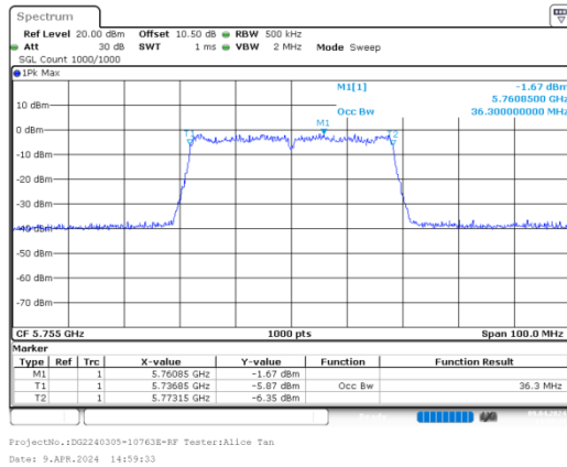
n40_5755MHz_Chain 0
