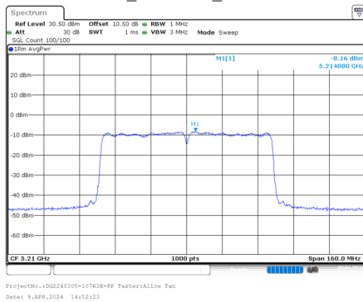
ac80_5210MHz_Chain 0
