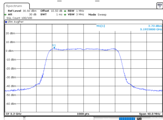
ac20_5200MHz_Chain 1
