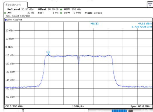
n40_5755MHz_Chain 1
