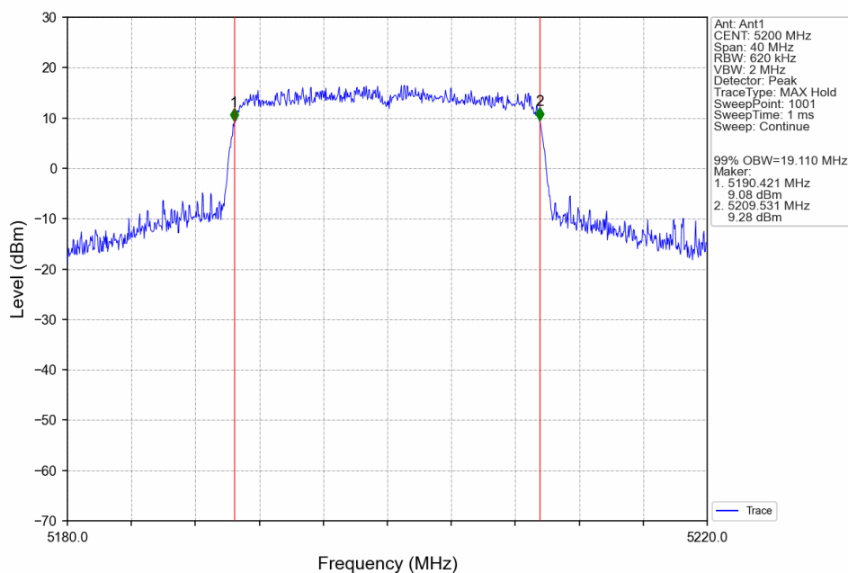
802.11be(EHT20)_MCH_5200MHz_SU_ / _Ant1_NTNV
