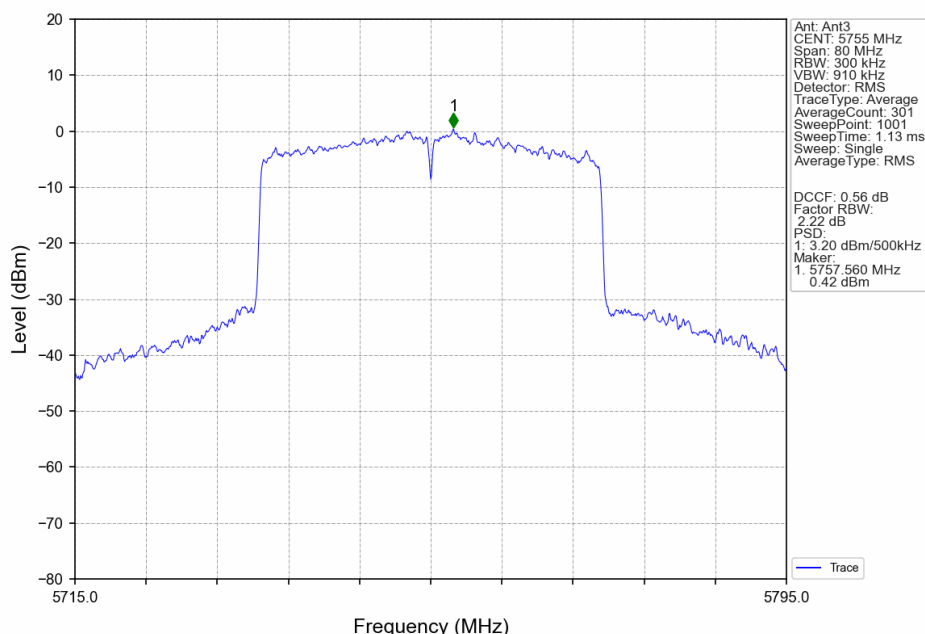
802.11be(EHT40)_LCH_5755MHz_SU_/_Ant3_NTNV
