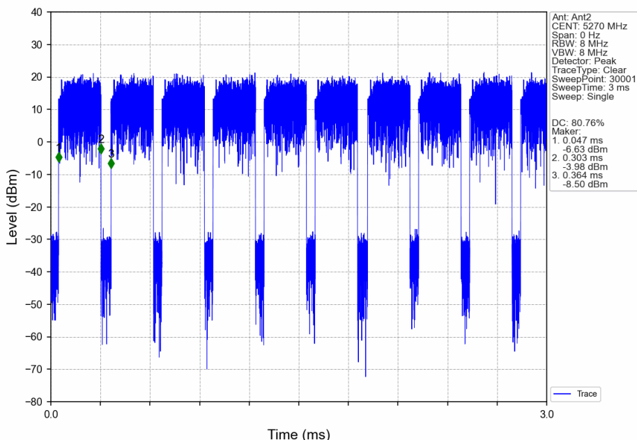
802.11ac(VHT40)_LCH_5270MHz_Ant2_NTNV
