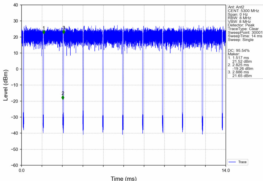
802.11n(HT20)_MCH_5300MHz_Ant2_NTNV
