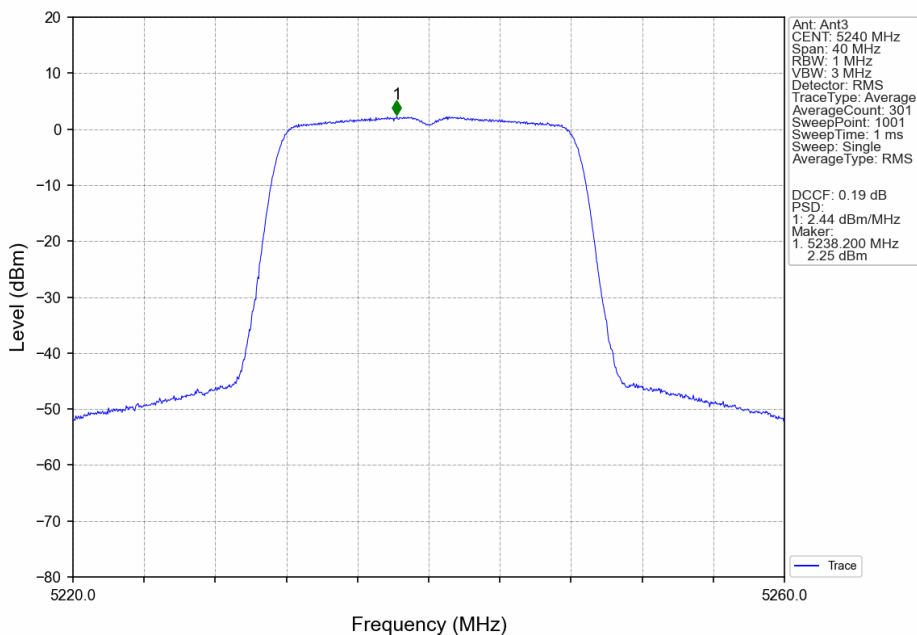
802.11a_HCH_5240MHz_Ant3_NTNV
