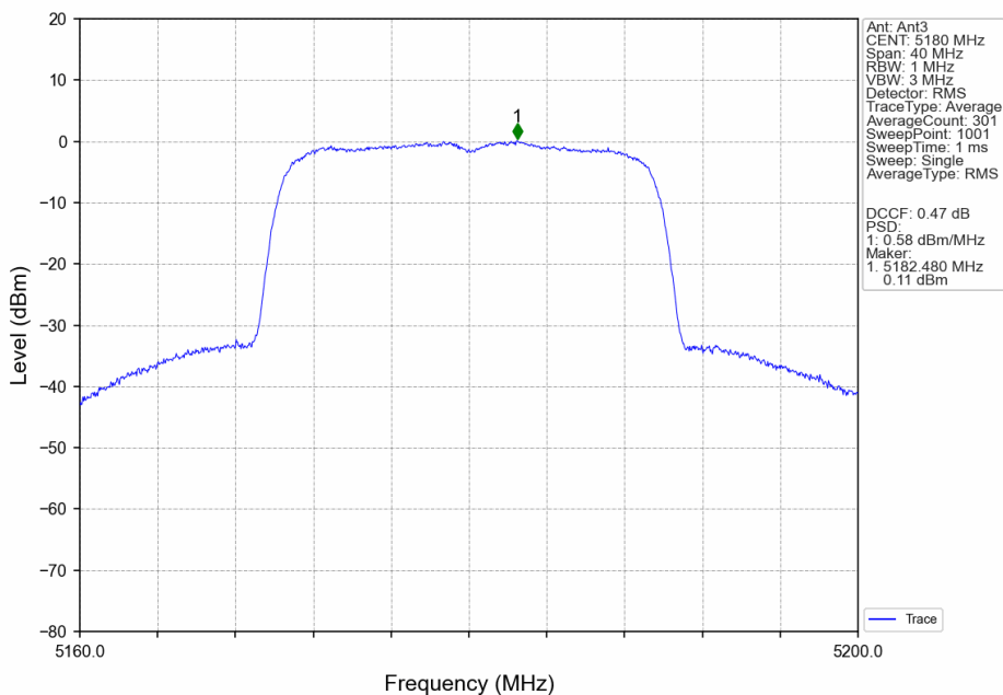
802.11be(EHT20)_LCH_5180MHz_SU_/_Ant3_NTNV
