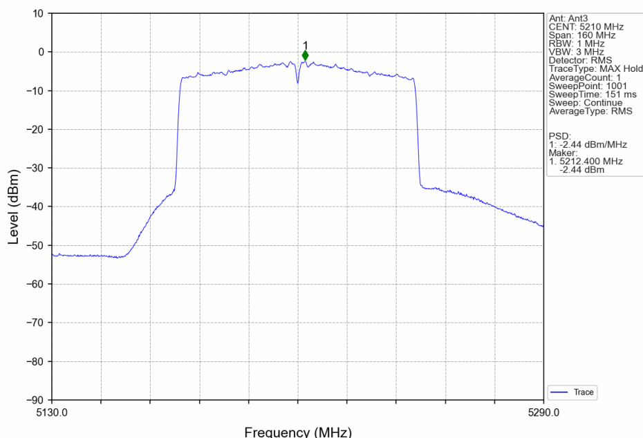
802.11ac(VHT80)_MCH_5210MHz_Ant3_NTNV
