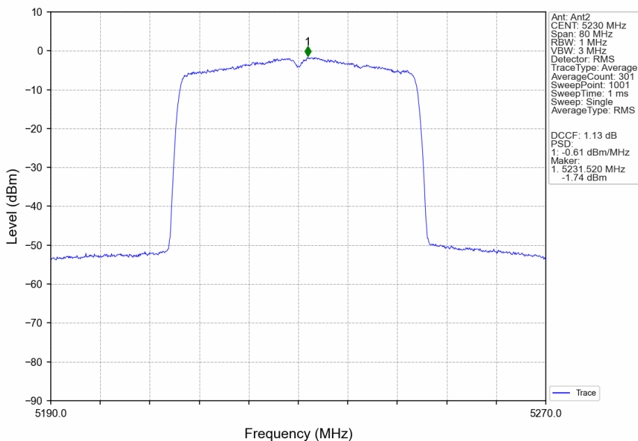
802.11be(EHT40)_HCH_5230MHz_SU_/_Ant2_NTNV
