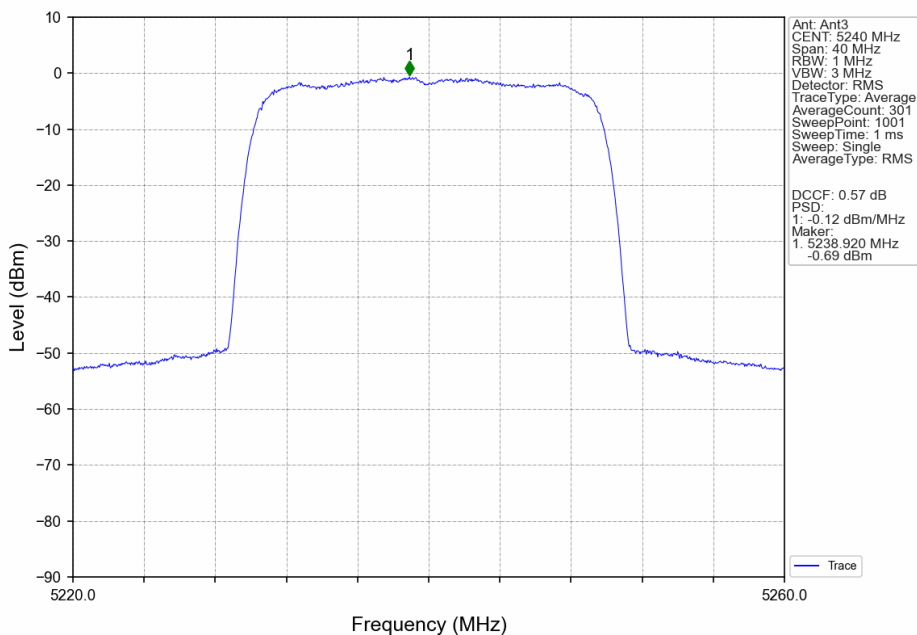
802.11be(EHT20)_HCH_5240MHz_SU_ / _Ant3_NTNV
