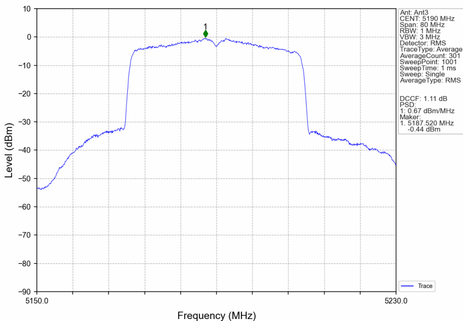
802.11be(EHT40)_LCH_5190MHz_SU_ / _Ant3_NTNV
