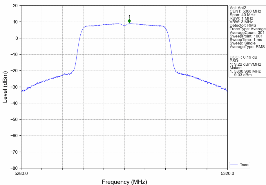
802.11a_MCH_5300MHz_Ant2_NTNV
