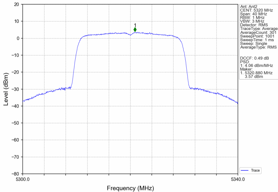
802.11be(EHT20)_HCH_5320MHz_SU_/_MIMO_NTNV
