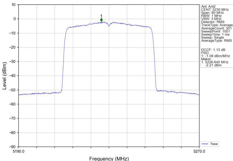
802.11be(EHT40)_HCH_5230MHz_SU_/_MIMO_NTNV
