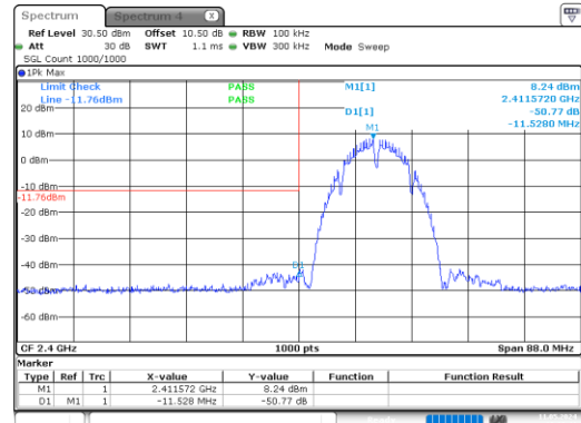
b_2412MHz_Chain 1
