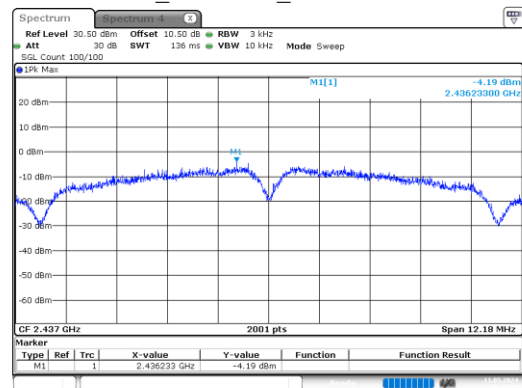
b_2437MHz_Chain 1
