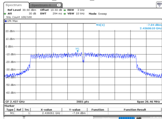
n20_2437MHz_Chain 1
