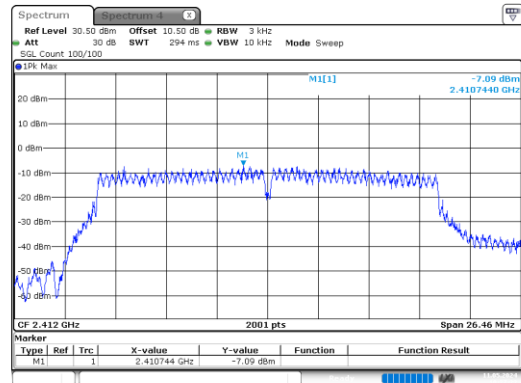
n20_2412MHz_Chain 1
