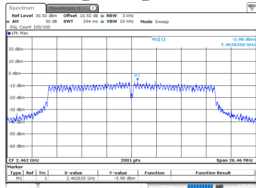
n20_2462MHz_Chain 1
