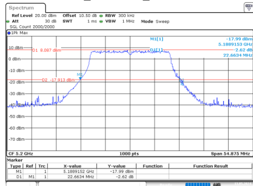
ac20_5200MHz_Chain 0
