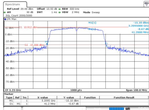
n40_5230MHz_Chain 0
