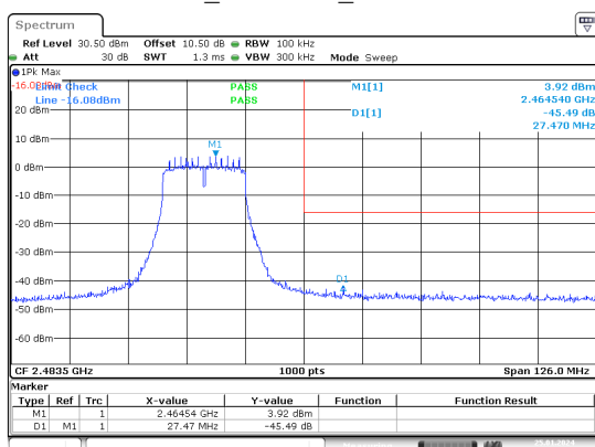
n20_2462MHz_Chain 0
