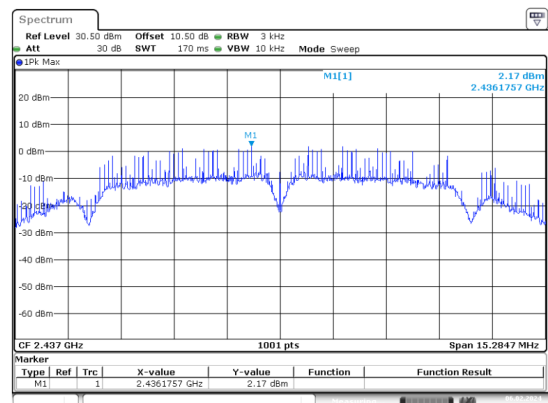
b_2437MHz_Chain 1
