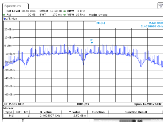
b_2462MHz_Chain 0
