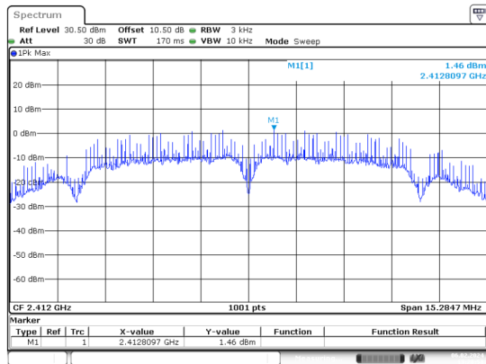
b_2412MHz_Chain 0
