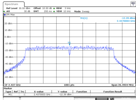
n20_2437MHz_Chain 1
