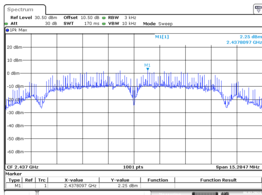
b_2437MHz_Chain 0
