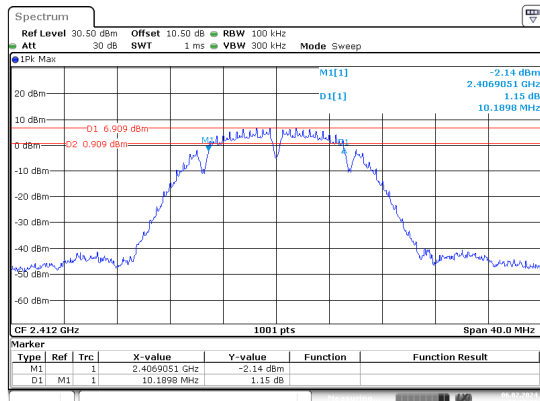
b_2412MHz_Chain 0
