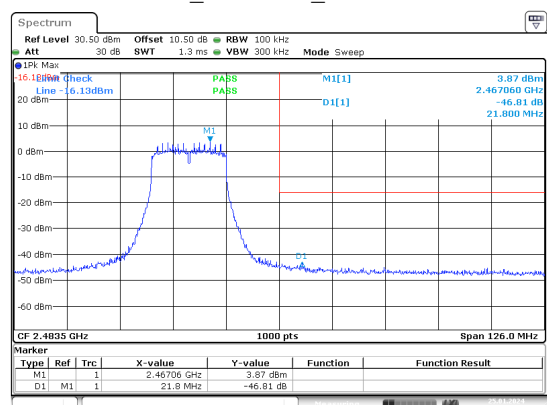
n20_2462MHz_Chain 1
