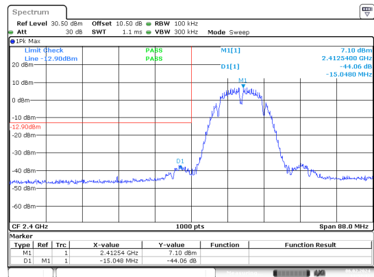
b_2412MHz_Chain 1
