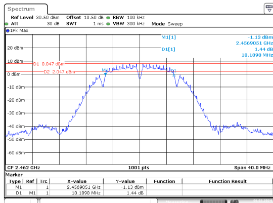
b_2462MHz_Chain 0
