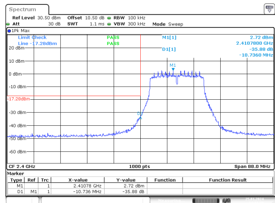
n20_2412MHz_Chain 1
