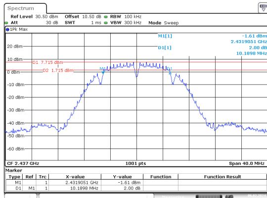
b_2437MHz_Chain 0
