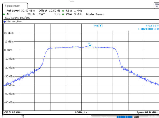
ac20_5180MHz
