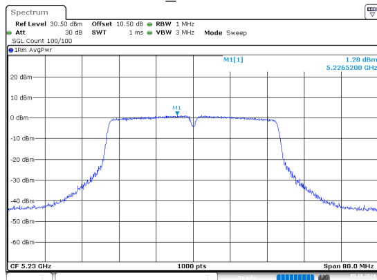
ac40_5230MHz
