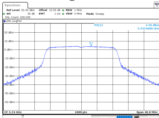
ac20_5240MHz
