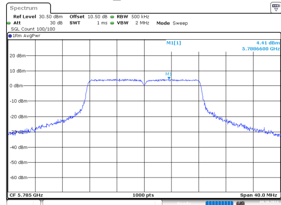
a_5785MHz
