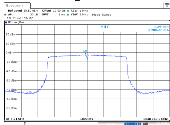
ac80_5210MHz
