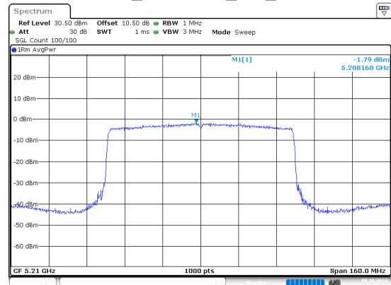
ax80_5210MHz_RU_Full
