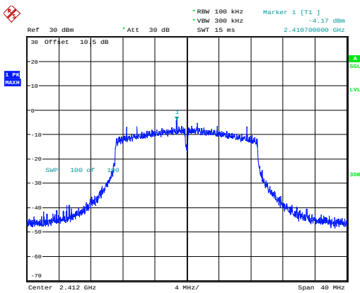
802.11n20_2412MHz_Chain 1
