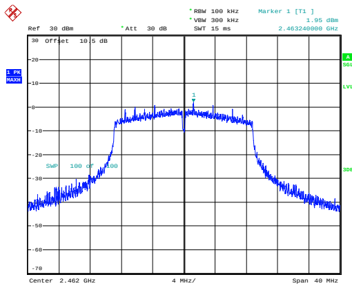
802.11n20_2462MHz_Chain 0
