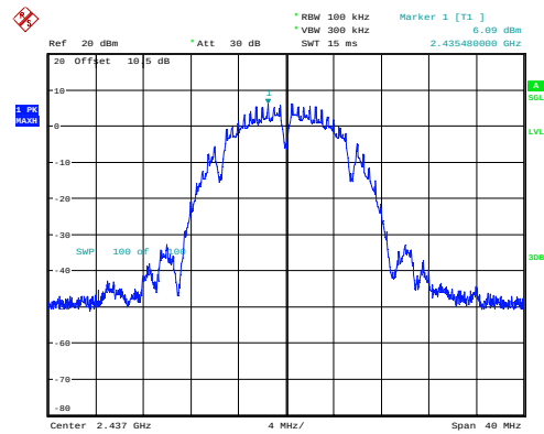
802.11b_2437MHz_Chain 0
