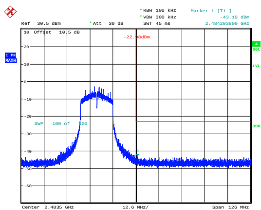
802.11n20_2462MHz_Chain 1
