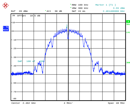
802.11b_2462MHz_Chain 1
