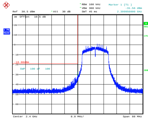
802.11n20_2412MHz_Chain 0
