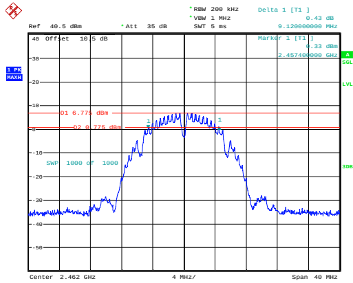
802.11b_2462MHz_Chain 0
