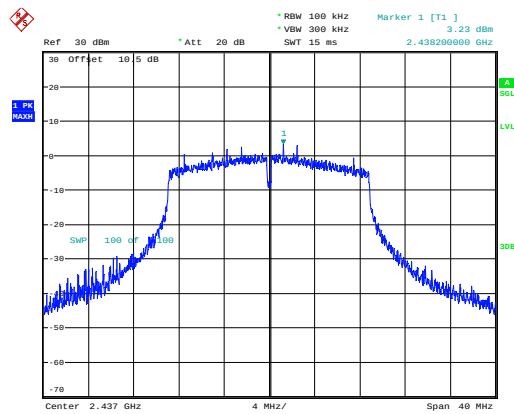
802.11n20_2437MHz_Chain 0
