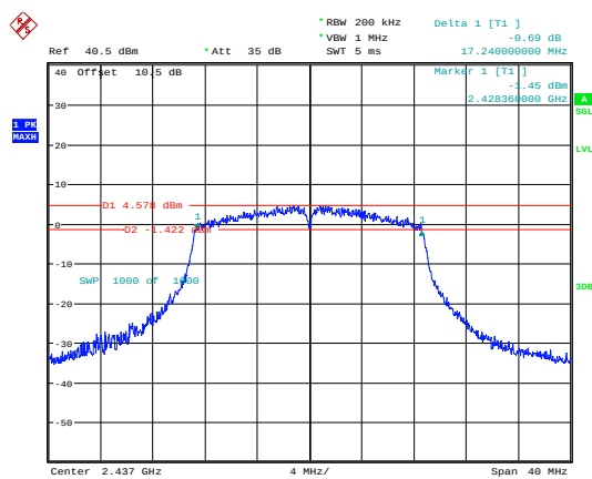
802.11n20_2437MHz_Chain 0
