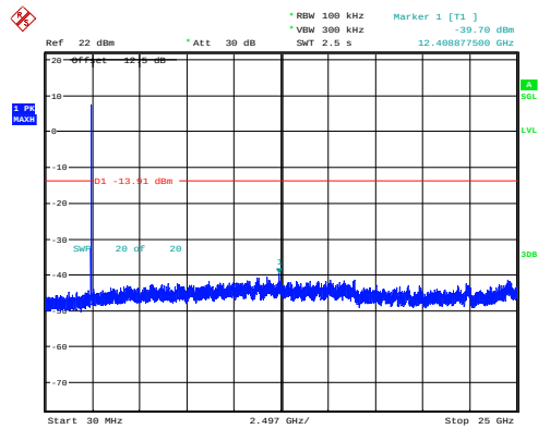
802.11b_2437MHz_Chain 0
