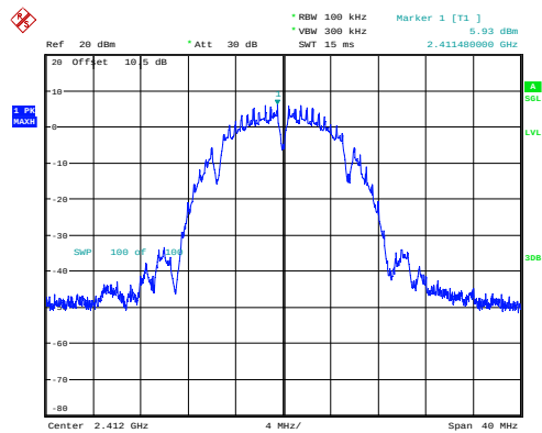
802.11b_2412MHz_Chain 0
