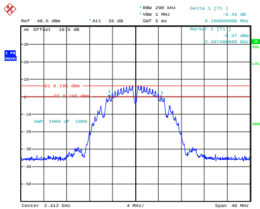
802.11b_2412MHz_Chain 0
