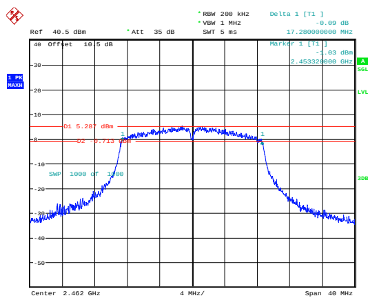
802.11n20_2462MHz_Chain 0
