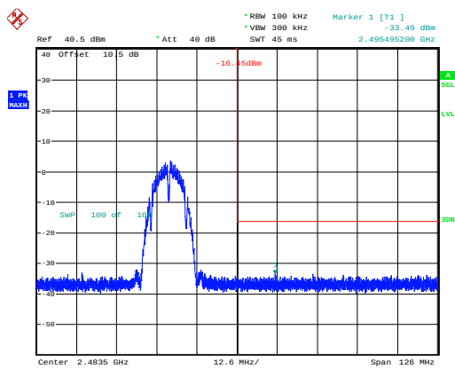
802.11b_2462MHz_Chain 1
