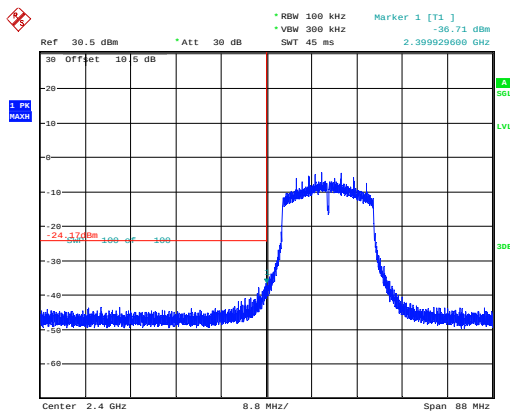
802.11n20_2412MHz_Chain 1
