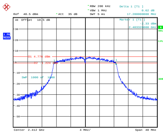
802.11n20_2412MHz_Chain 0
