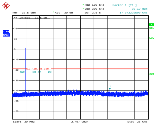
802.11n20_2412MHz_Chain 0
