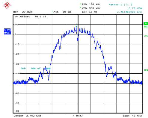
802.11b_2462MHz_Chain 0
