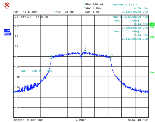
802.11n20_2437MHz_Chain 0
