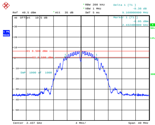
802.11b_2437MHz_Chain 0
