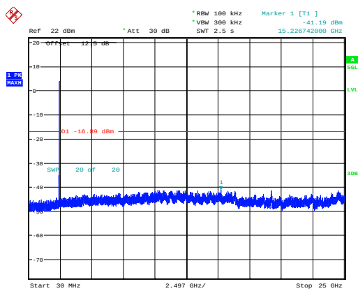
802.11b_2437MHz_Chain 1
