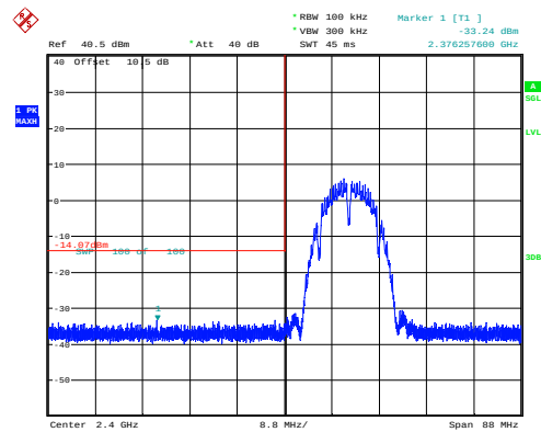
802.11b_2412MHz_Chain 0
