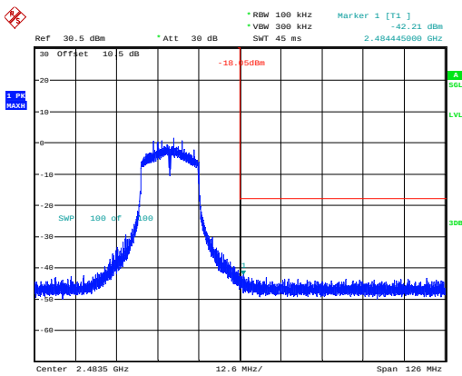
802.11n20_2462MHz_Chain 0
