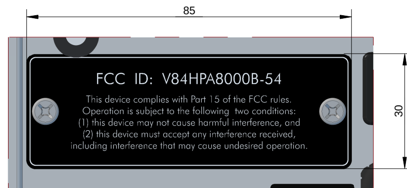
Detail A 1:1
