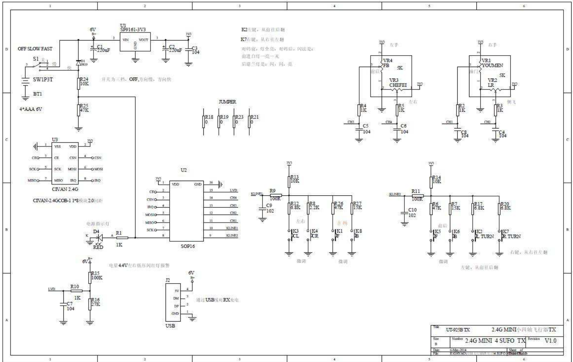
236TX微調自轉電路圖 (1177x759x16M png)
