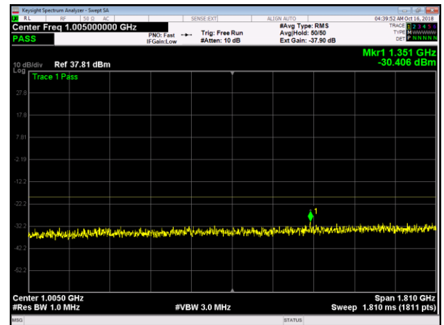
Band 25, LTE10, B, Upper, 100MHz-1910MHz
