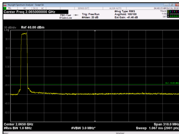
Band 25, LTE10, B, Upper, 1910MHz-2220MHz
