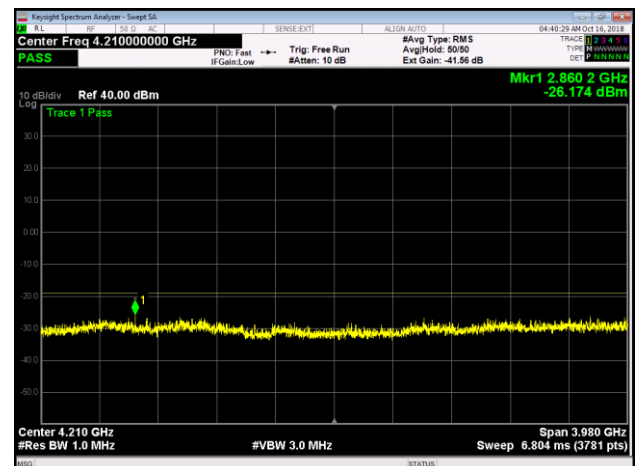
Band 25, LTE10, B, Upper, 2220MHz-6200MHz
