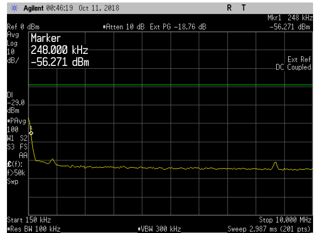
Band 25, LTE10, B, Upper, 150KHz-10MHz
