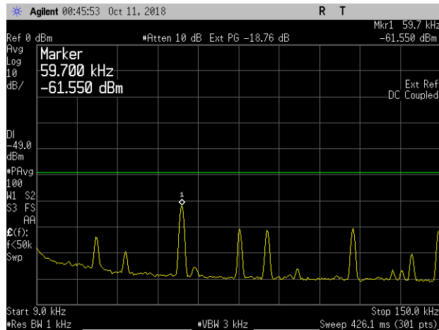
Band 25, LTE10, B, Upper, 9KHz-150KHz
