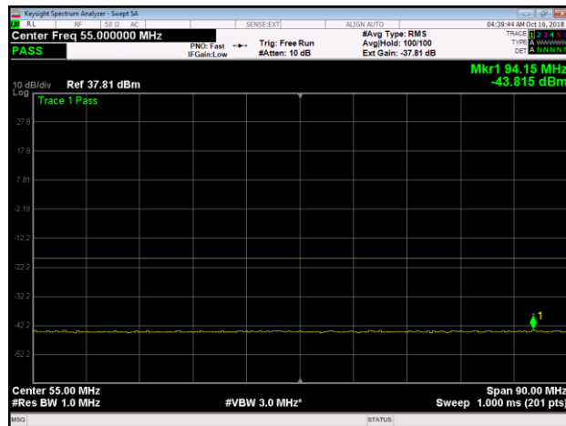
Band 25, LTE10, B, Upper, 10MHz-100MHz
