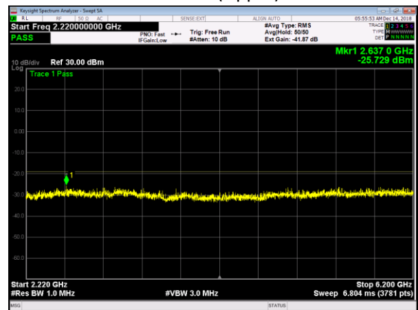
LTE15 Middle+NB IoT GB (Upper) 2220MHz-6.2GHz
