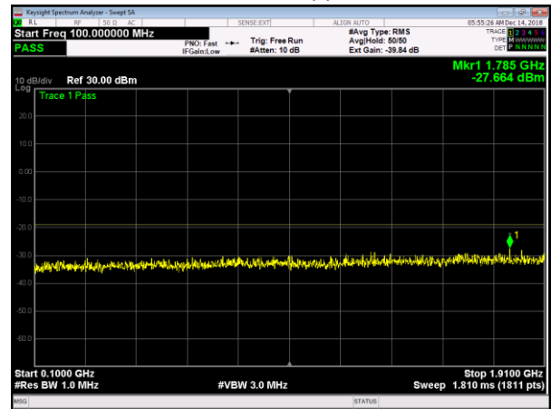
LTE15 Middle+NB IoT GB (Upper) 100MHz-1910MHz
