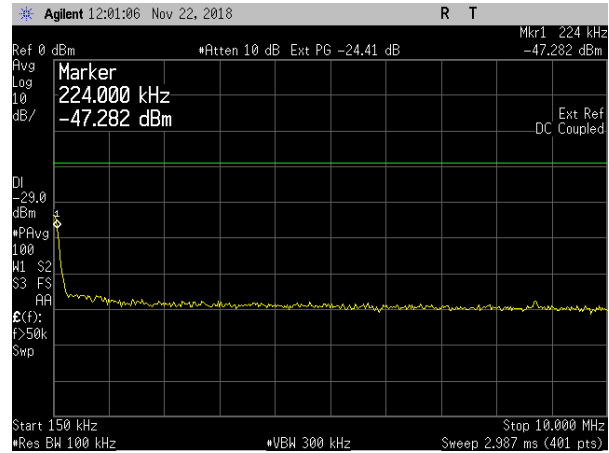
LTE15 Bottom+NB IoT GB (Upper) 150KHz-10MHz
