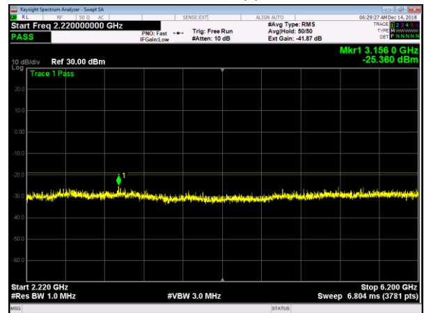
LTE15 Bottom+NB IoT GB (Upper) 2220MHz-6.2GHz
