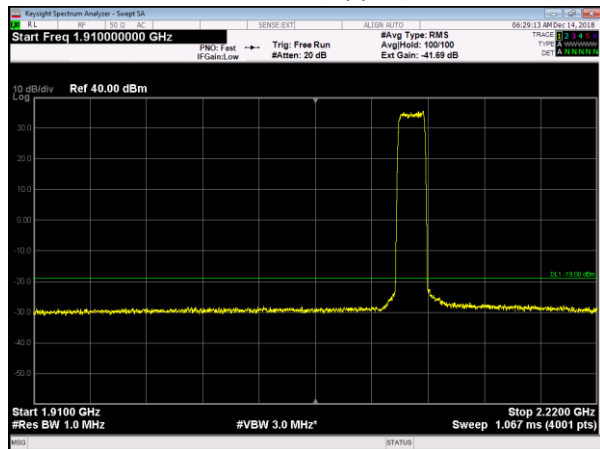
LTE15 Bottom+NB IoT GB (Upper) 1910MHz-2220MHz
