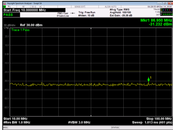
LTE15 Bottom+NB IoT GB (Upper) 10MHz-100MHz
