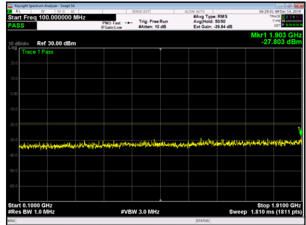
LTE15 Bottom+NB IoT GB (Upper) 100MHz-1910MHz
