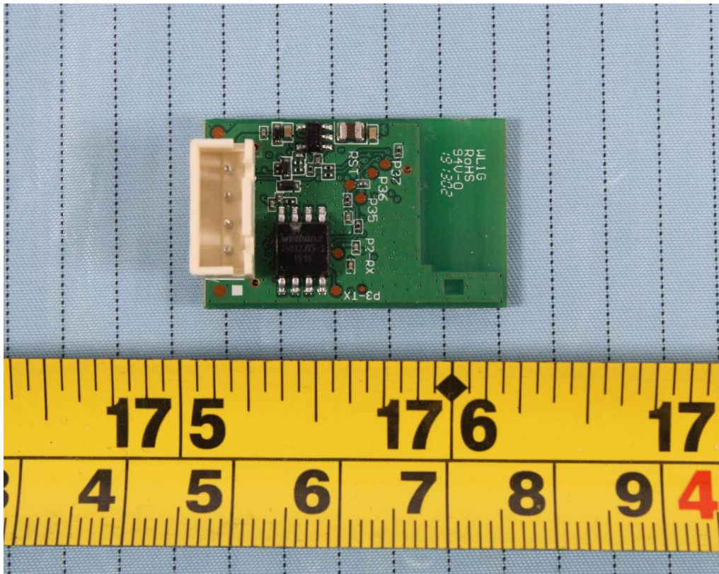
Wi-Fi Module
