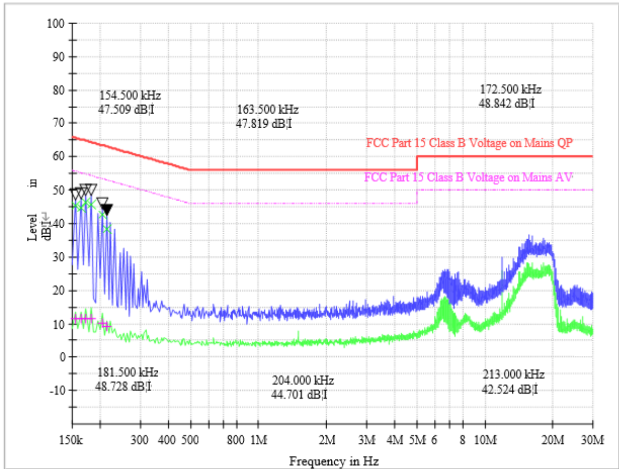
(Plot E: L1 Phase)
