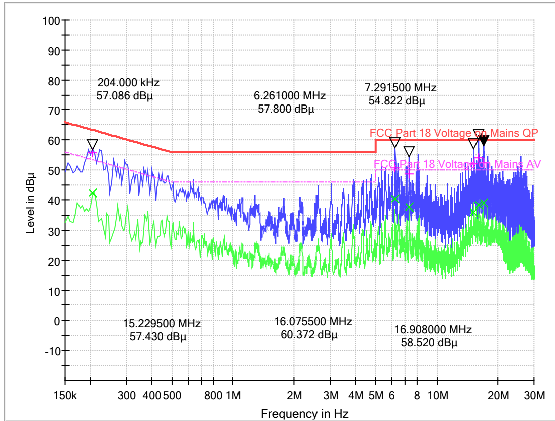
(Plot A: L1 Phase)
