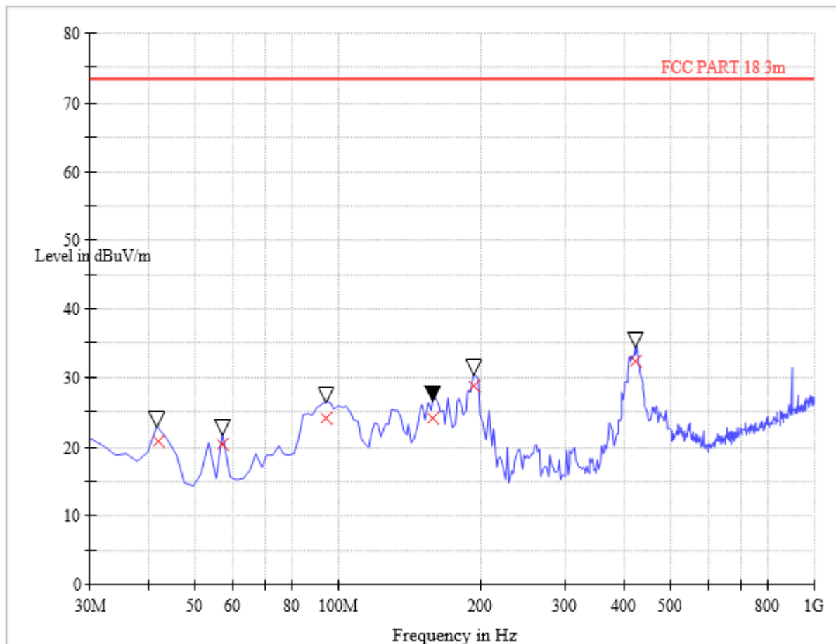
(Plot A: Test Antenna Horizontal 30M - 1G)
