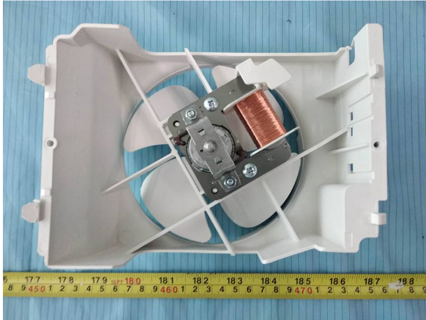
EUT – Exhaust Fan Bottom View
