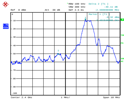
Port 1, 2400 MHz Band Edge
