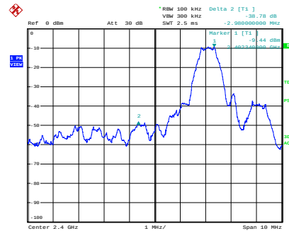
Port 2, 2400 MHz Band Edge
