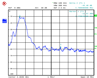
Port 1, 2483.5 MHz Band Edge
