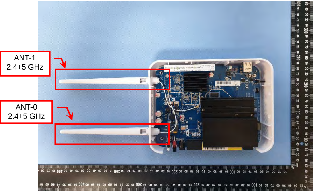
EUT Photo (2)
