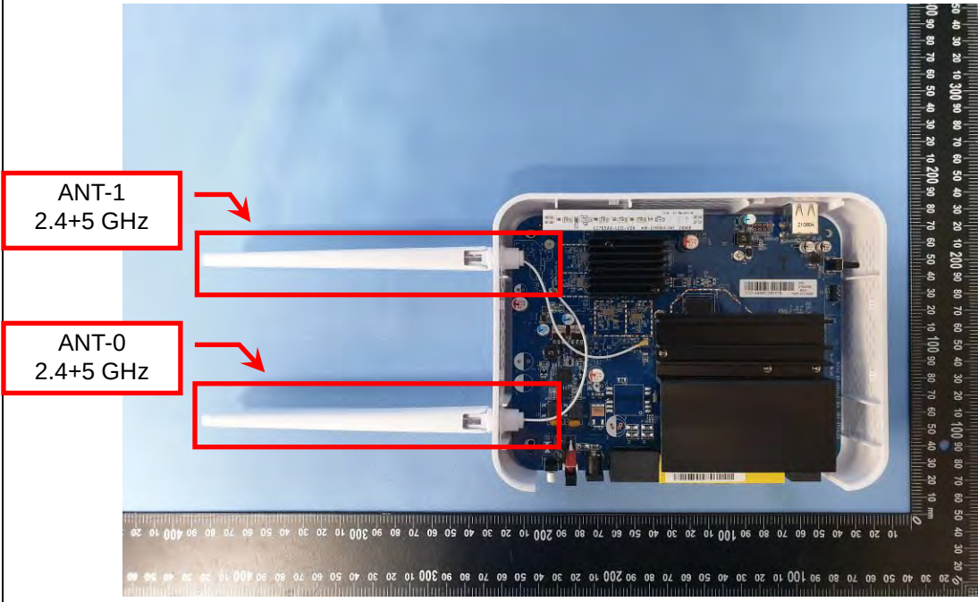
EUT Photo (2)
