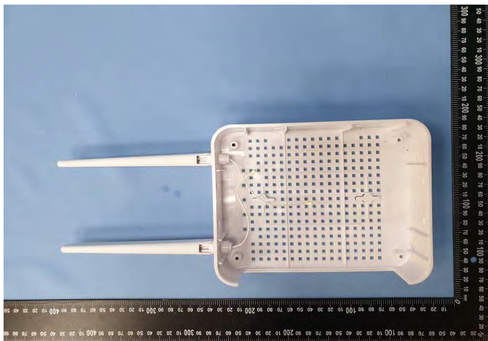
EUT Photo (21)
