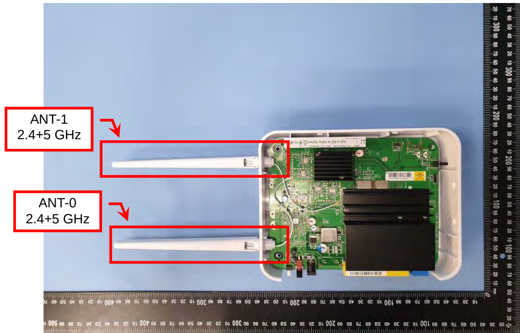
EUT Photo (2)
