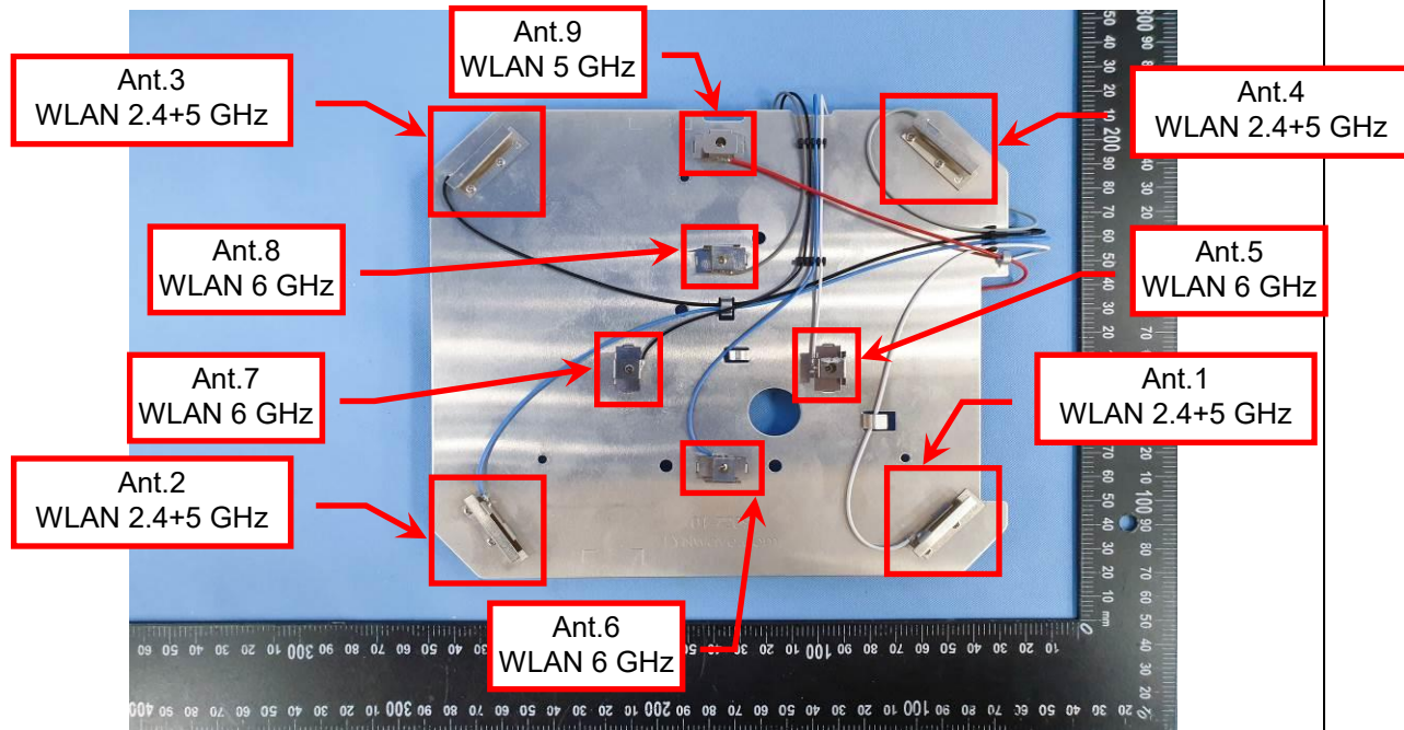
EUT Photo (4)
