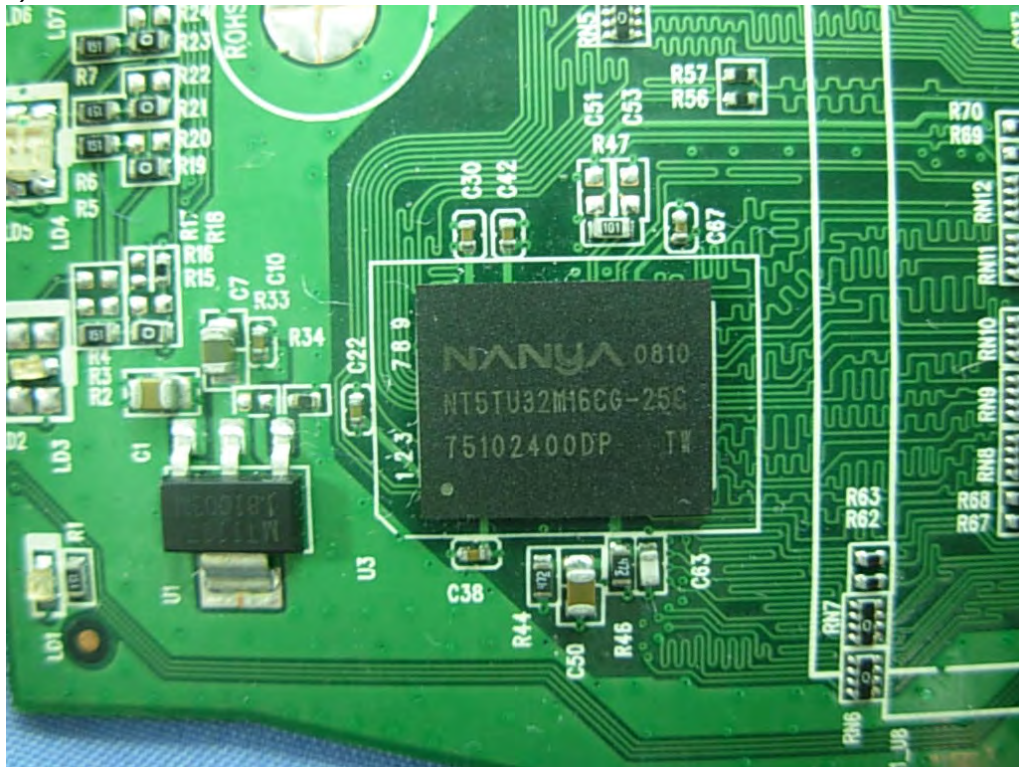
(17) EUT Photo
