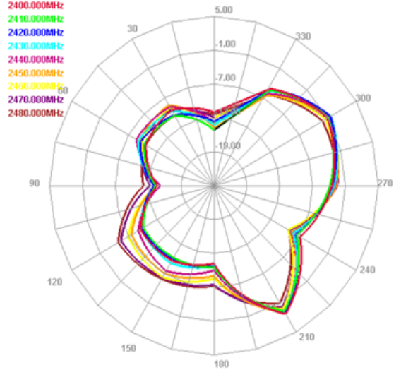
2480.000MHz
