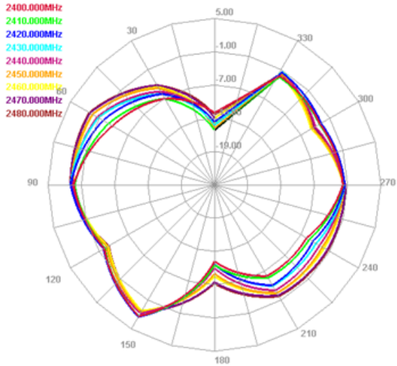
2450.000MHz
