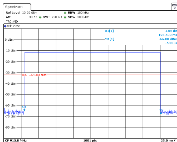
2FSK (38.4 kbps)
