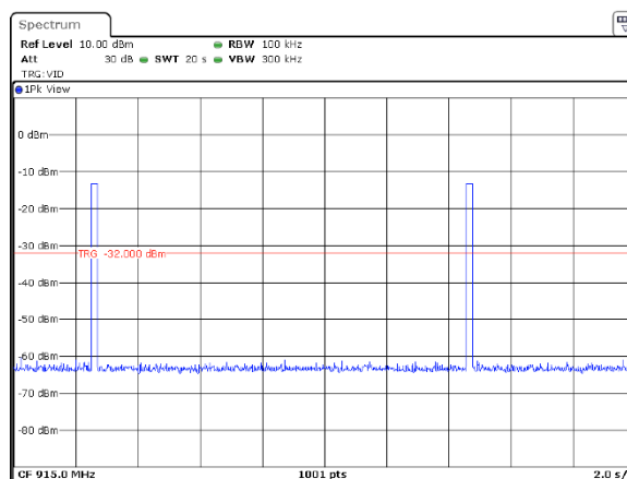
GFSK (50 kbps)
