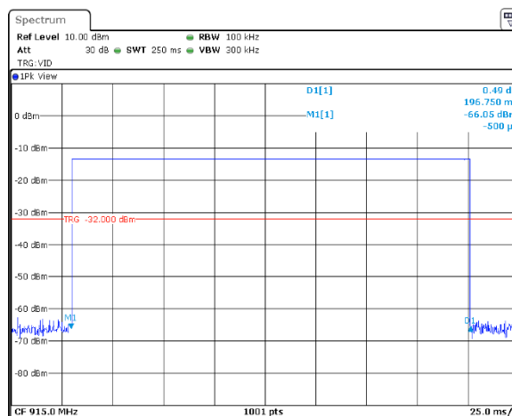
GFSK (50 kbps)
