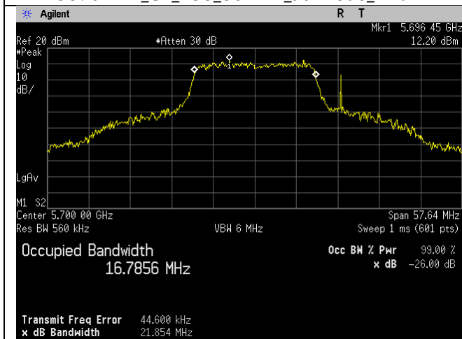
5700MHz_Ch_140_20MHz_a-mode_Ant A
