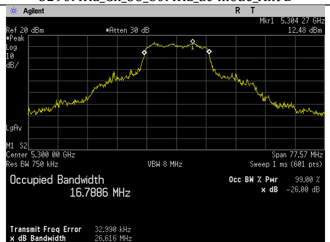
5300MHz_Ch_60_20MHz_a-mode_Ant B
