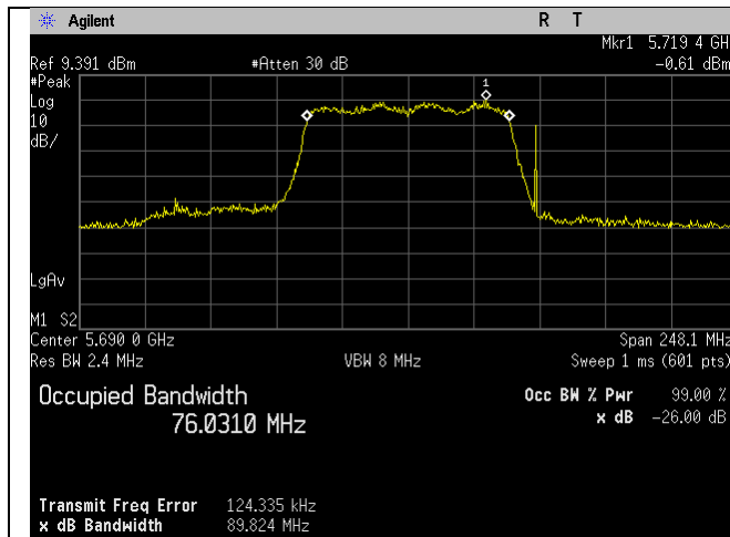
5690MHz_138_80MHz_ac-mode_Ant C
