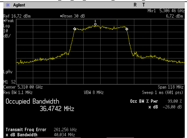
5310MHz_Ch_62_40MHz_n-mode_Ant B
