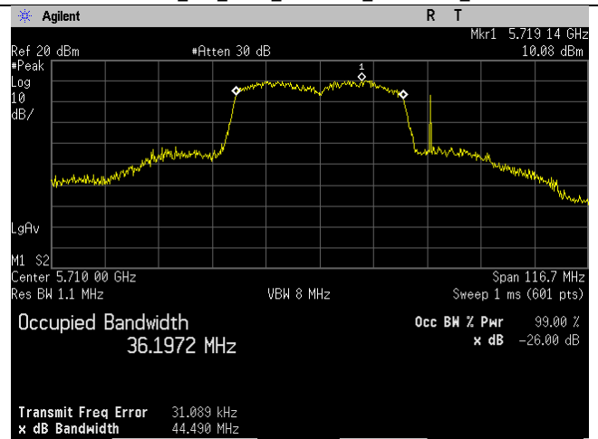
5710MHz_Ch_142_40MHz_n-mode_Ant B
