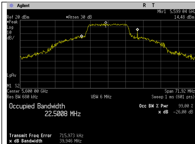
5600MHz_Ch_120_20MHz_a-mode_Ant A
