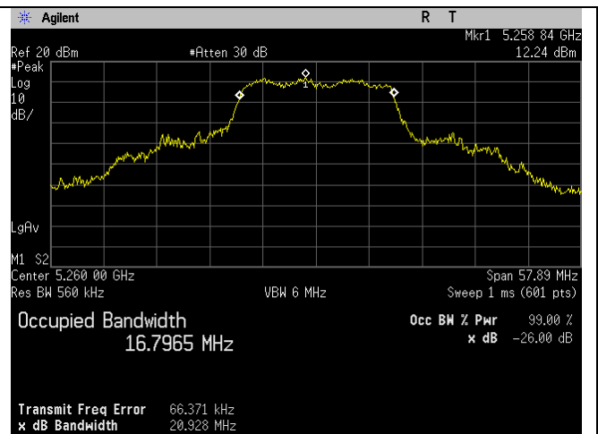
5260MHz_Ch_52_20MHz_a-mode_Ant B
