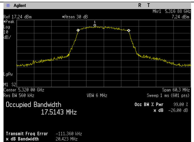
5320MHz_Ch_64_20MHz_n-mode_Ant B
