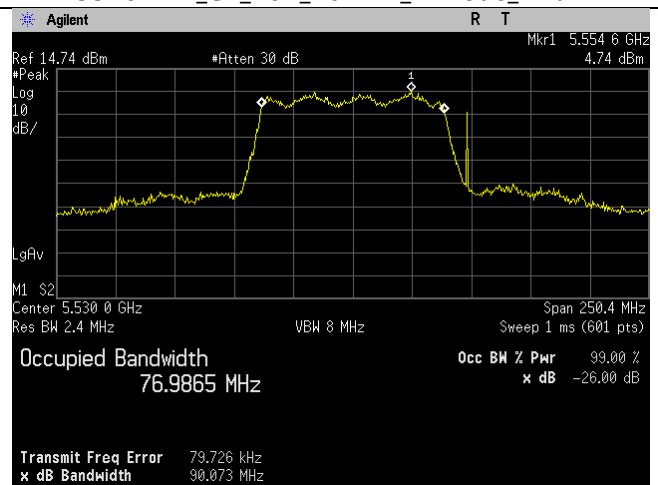
5530MHz_Ch_106_80MHz_ac-mode_Ant B
