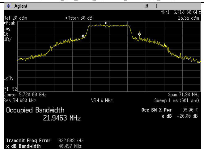
5720MHz_Ch_144_20MHz_a-mode_Ant B
