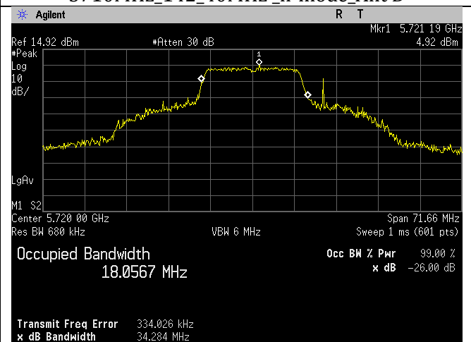
5720MHz_144_20MHz_a-mode_Ant D
