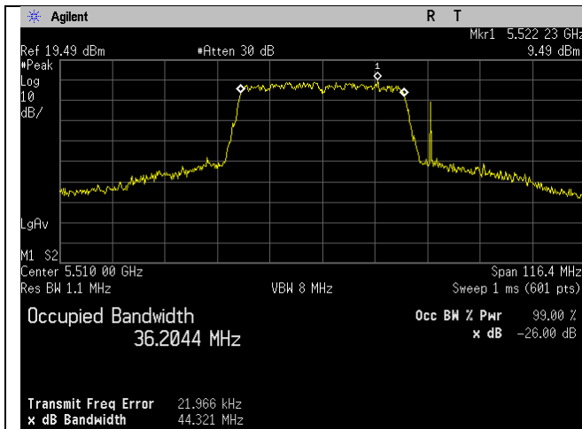
5510MHz_Ch_102_40MHz_n-mode_Ant A
