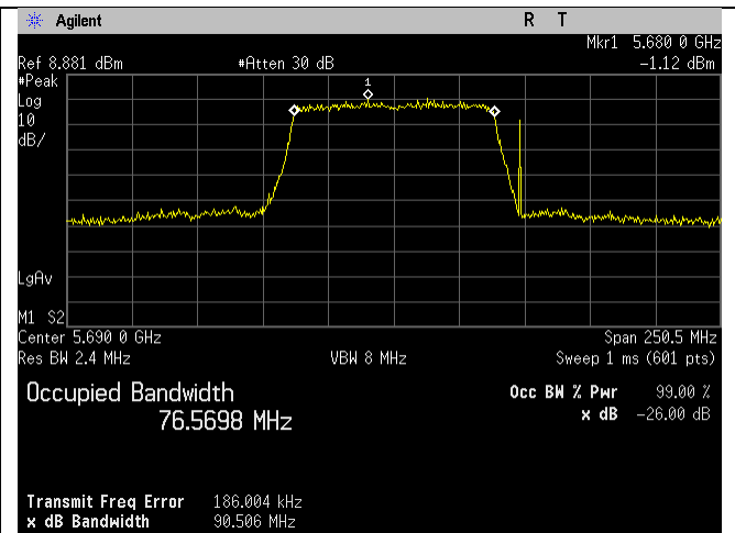
5690MHz_138_80MHz_ac-mode_Ant D
