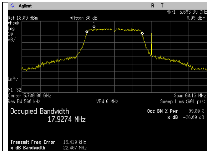
5700MHz_Ch_140_20MHz_n-mode_Ant A
