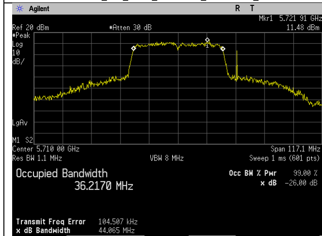
5710MHz_Ch_142_40MHz_n-mode_Ant A
