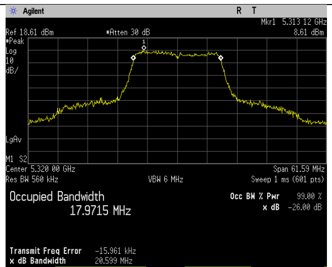
5320MHz_64_20MHz_n-mode_Ant D
