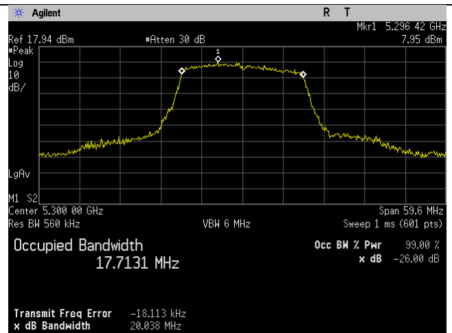
5300MHz_Ch_60_20MHz_n-mode_Ant B
