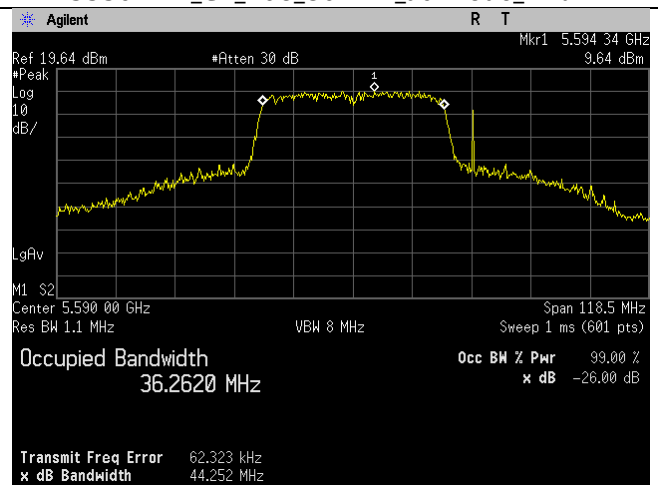
5590MHz_Ch_118_40MHz_n-mode_Ant B
