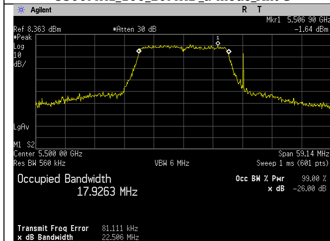
5500MHz_100_20MHz_n-mode_Ant C
