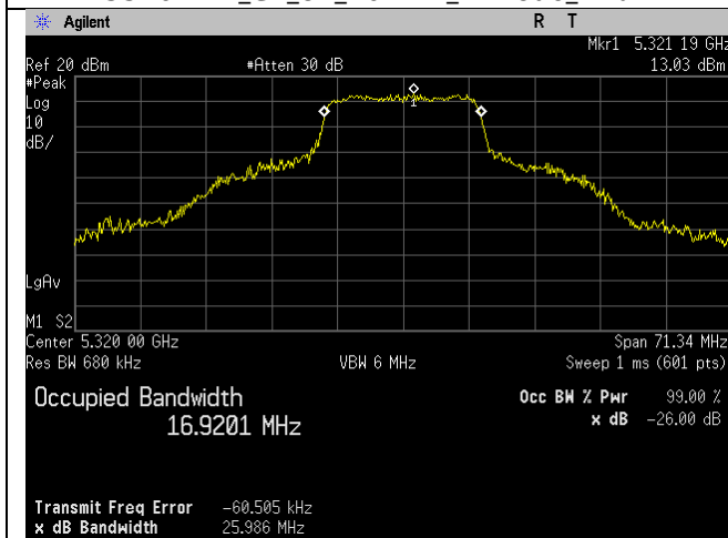
5320MHz_Ch_64_20MHz_a-mode_Ant A
