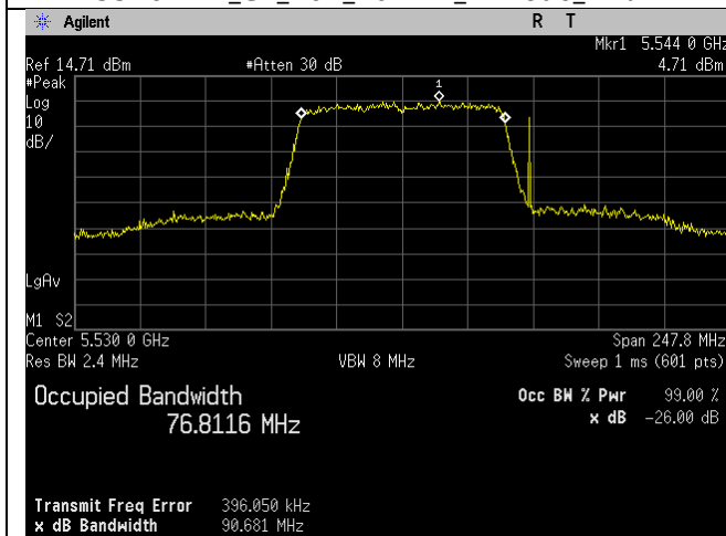
5530MHz_Ch_106_80MHz_ac-mode_Ant A
