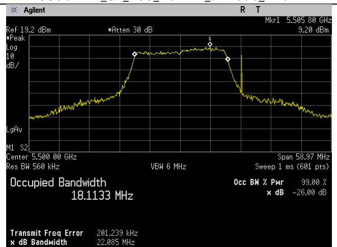
5500MHz_Ch_100_20MHz_n-mode_Ant B
