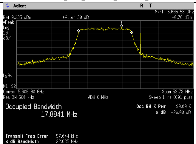
5600MHz_120_20MHz_n-mode_Ant D
