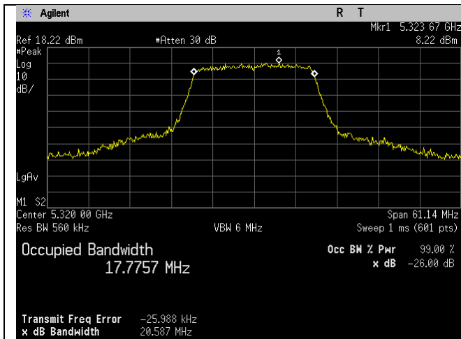
5320MHz_Ch_64_20MHz_n-mode_Ant A
