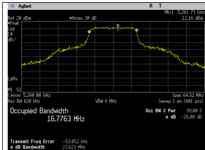
5260MHz_Ch_52_20MHz_a-mode_Ant A
