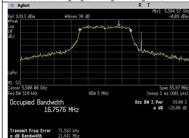
5500MHz_100_20MHz_a-mode_Ant C
