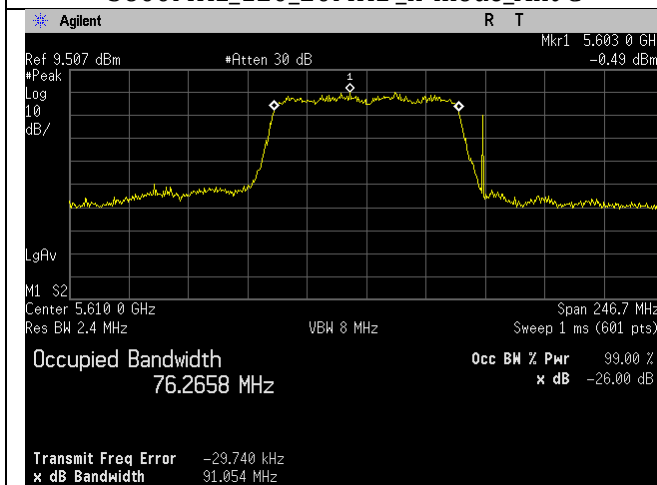
5610MHz_122_80MHz_ac-mode_Ant C
