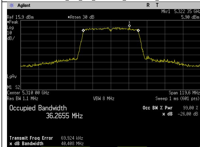
5310MHz_Ch_62_40MHz_n-mode_Ant A
