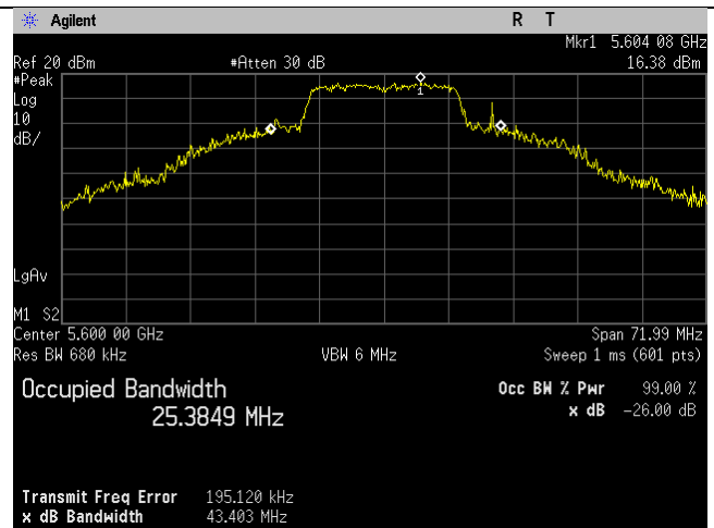
5600MHz_Ch_120_20MHz_a-mode_Ant B
