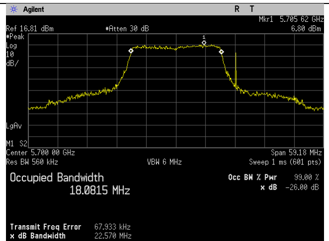
5700MHz_Ch_140_20MHz_n-mode_Ant B
