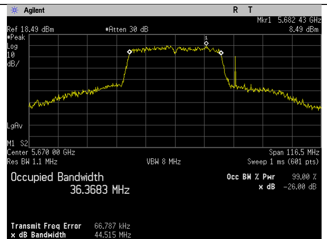
5670MHz_134_40MHz_n-mode_Ant D
