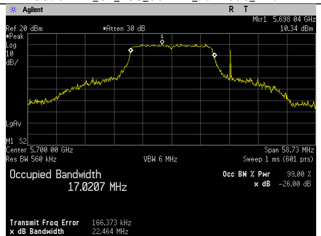
5700MHz_Ch_140_20MHz_a-mode_Ant B
