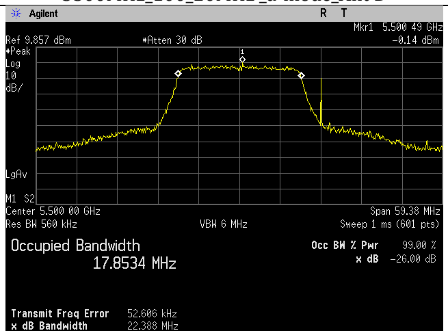
5500MHz_100_20MHz_n-mode_Ant D
