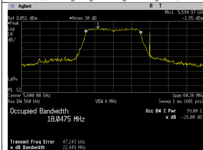
5600MHz_120_20MHz_n-mode_Ant C
