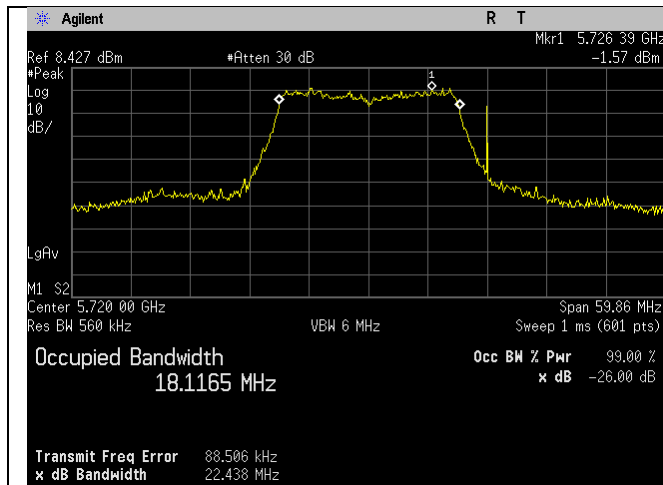
5720MHz_144_20MHz_n-mode_Ant C
