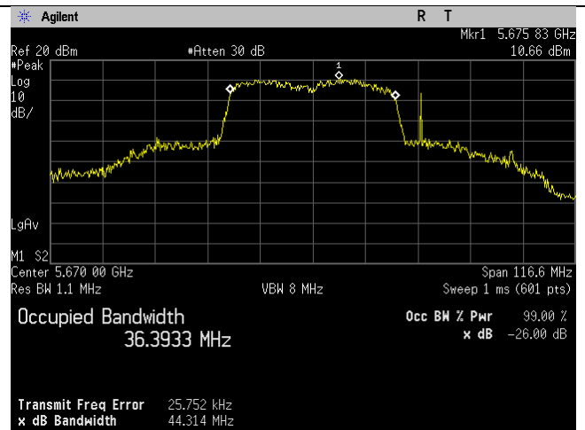
5670MHz_Ch_134_40MHz_n-mode_Ant B
