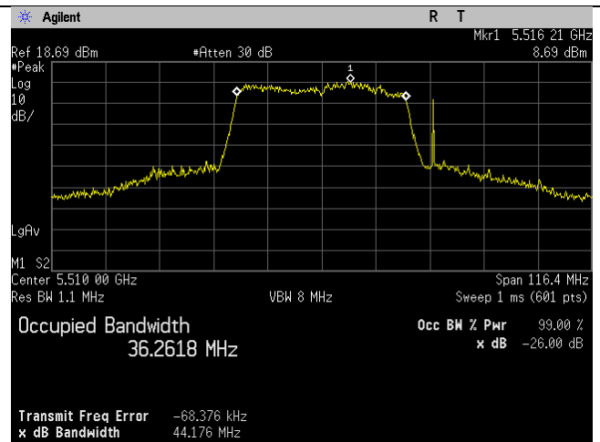
5510MHz_Ch_102_40MHz_n-mode_Ant B
