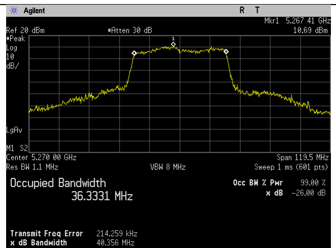
5270MHz_Ch_54_40MHz_n-mode_Ant B
