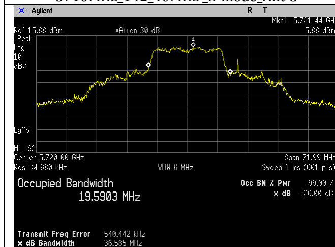
5720MHz_144_20MHz_a-mode_Ant C
