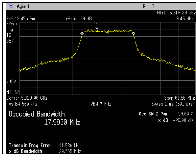
5320MHz_64_20MHz_n-mode_Ant C
