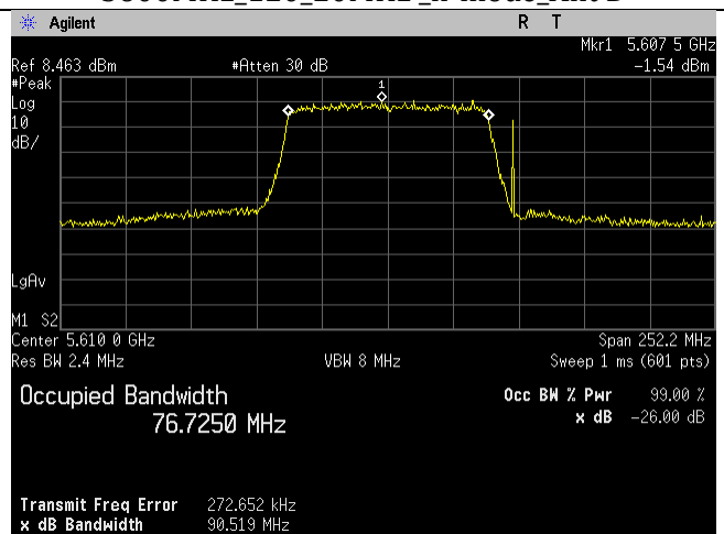
5610MHz_122_80MHz_ac-mode_Ant D
