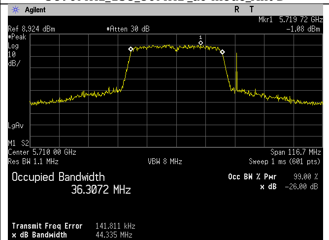
5710MHz_142_40MHz_n-mode_Ant D
