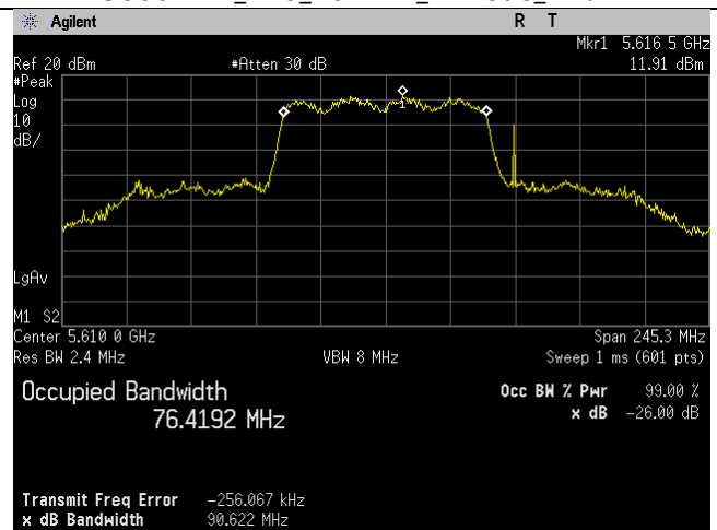
5610MHz_Ch_122_80MHz_ac-mode_Ant B
