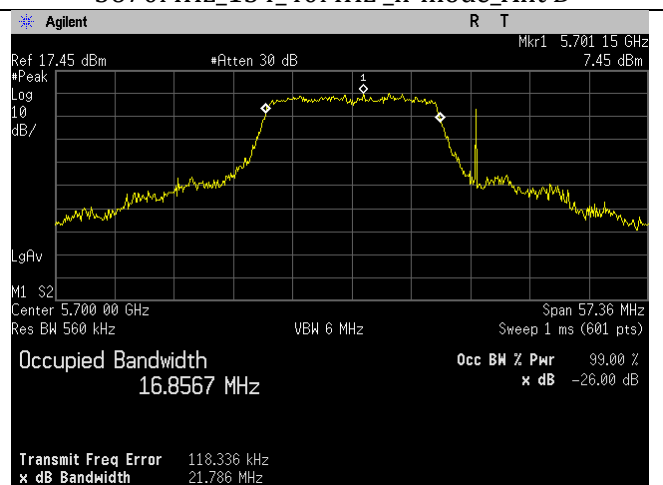
5700MHz_140_20MHz_a-mode_Ant D
