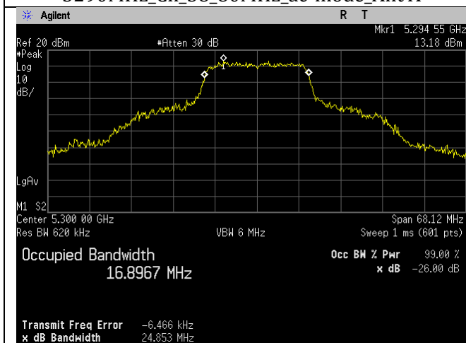
5300MHz_Ch_60_20MHz_a-mode_Ant A
