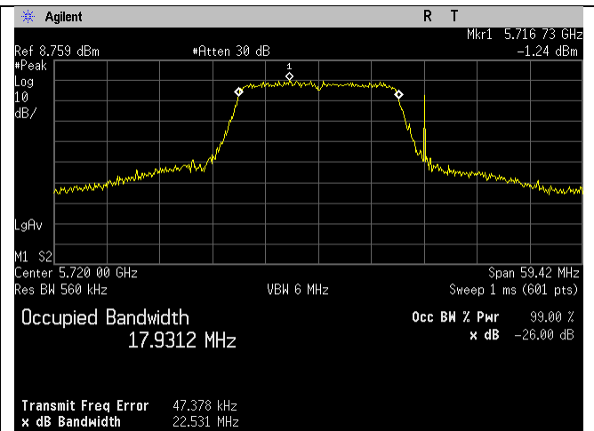
5720MHz_144_20MHz_n-mode_Ant D
