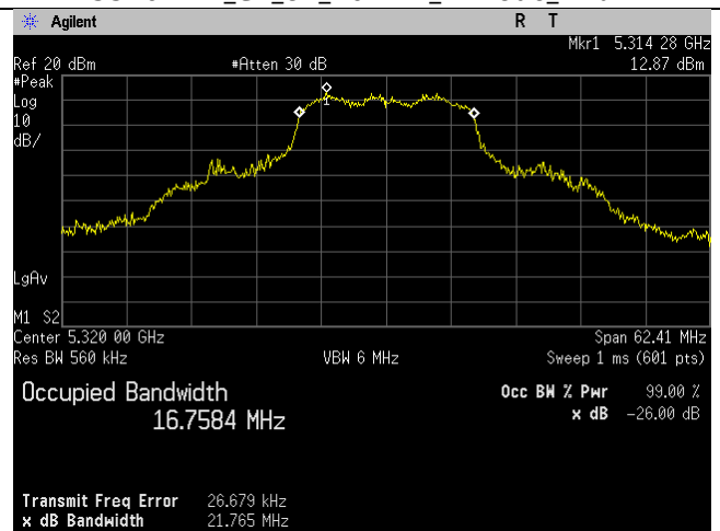
5320MHz_Ch_64_20MHz_a-mode_Ant B
