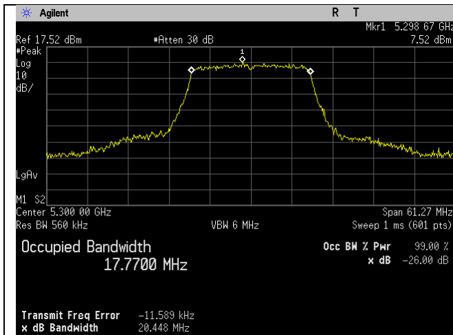
5300MHz_Ch_60_20MHz_n-mode_Ant A
