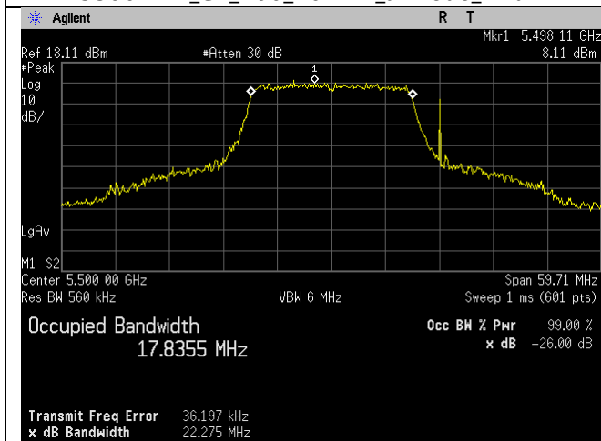
5500MHz_Ch_100_20MHz_n-mode_Ant A
