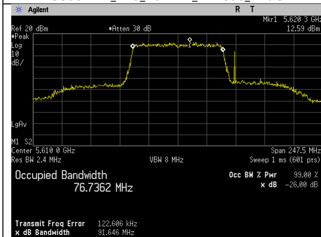
5610MHz_Ch_122_80MHz_ac-mode_Ant A
