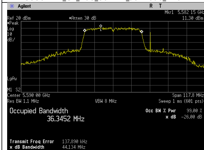
5590MHz_Ch_118_40MHz_n-mode_Ant A
