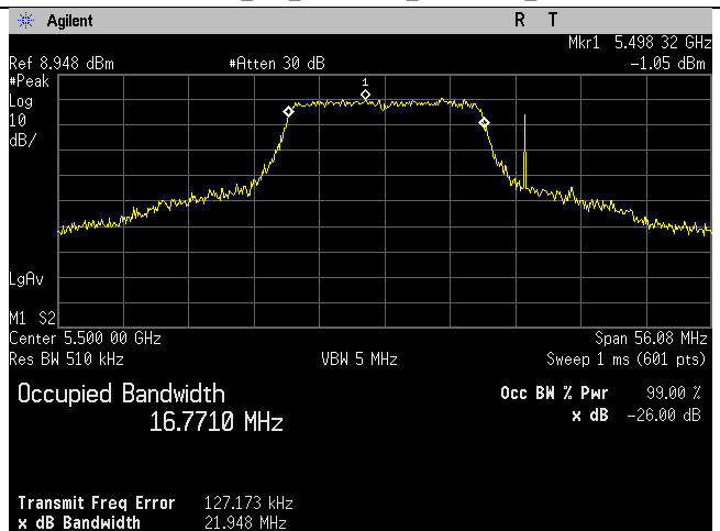
5500MHz_100_20MHz_a-mode_Ant D
