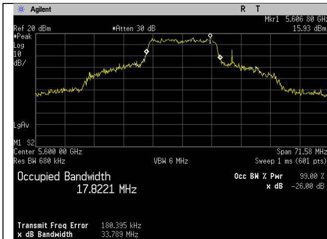
5600MHz_120_20MHz_a-mode_Ant C
