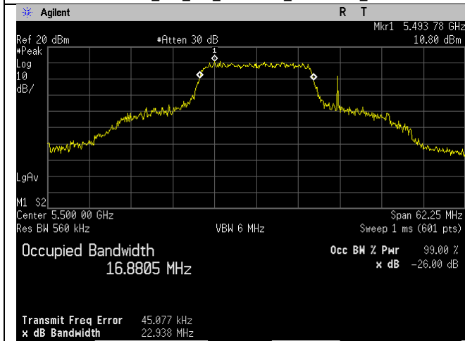
5500MHz_Ch_100_20MHz_a-mode_Ant A
