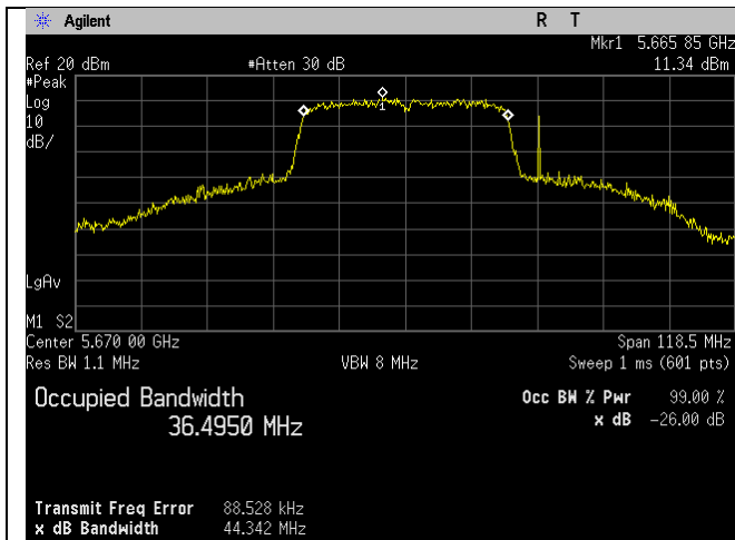
5670MHz_Ch_134_40MHz_n-mode_Ant A
