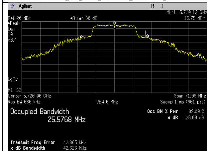
5720MHz_Ch_144_20MHz_a-mode_Ant A
