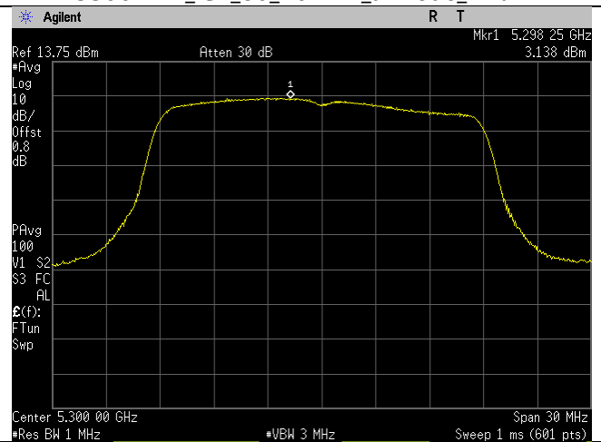
5300MHz_Ch_60_20MHz_n-mode_Ant B
