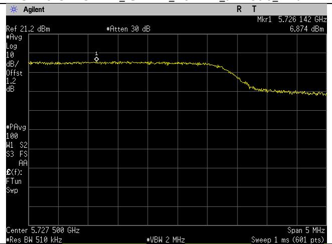
5725-5730MHz_Ch144_20MHz_a-mode Ant B
