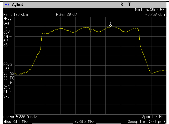
5290MHz_Ch_58_80MHz_ac-mode_Ant B
