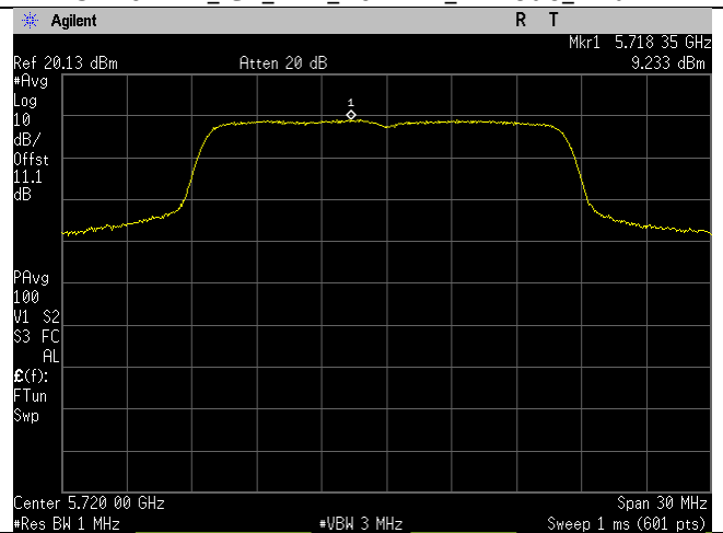
5720MHz_Ch_144_20MHz_a-mode Ant D
