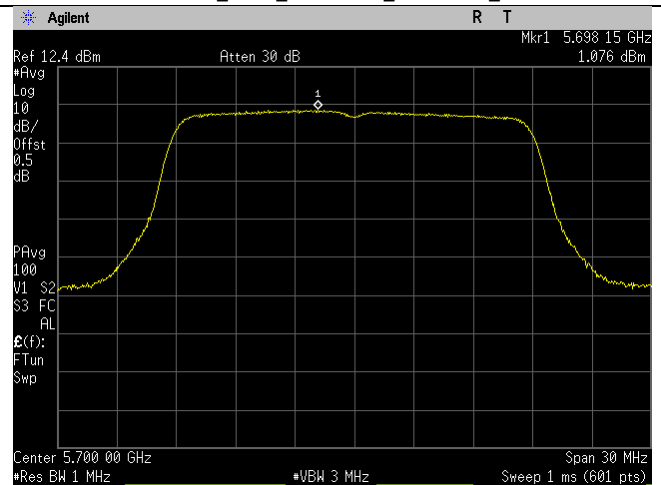
5700MHz_140_20MHz_n-mode_Ant D
