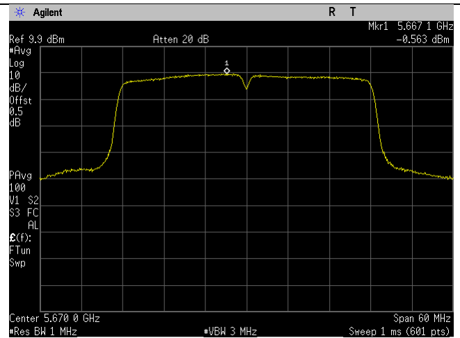
5670MHz_134_40MHz_n-mode_Ant D
