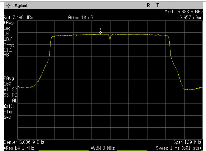
5690MHz_Ch_138_80MHz_ac-mode Ant D
