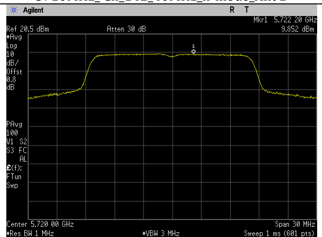
5720MHz_Ch_144_20MHz_a-mode_Ant B
