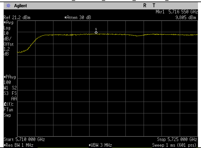
5710-5725MHz_Ch144_20MHz_a-mode Ant B
