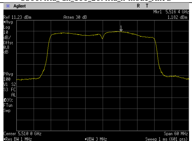
5510MHz_Ch_102_40MHz_n-mode_Ant B
