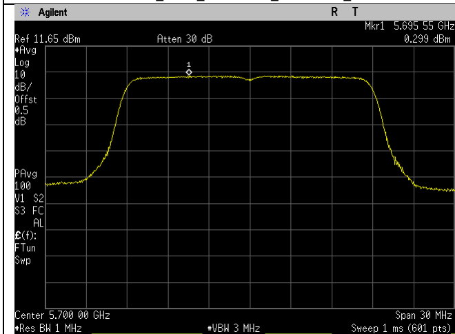
5700MHz_140_20MHz_n-mode_Ant C
