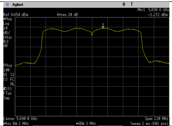
5690MHz_Ch_138_80MHz_ac-mode_Ant B
