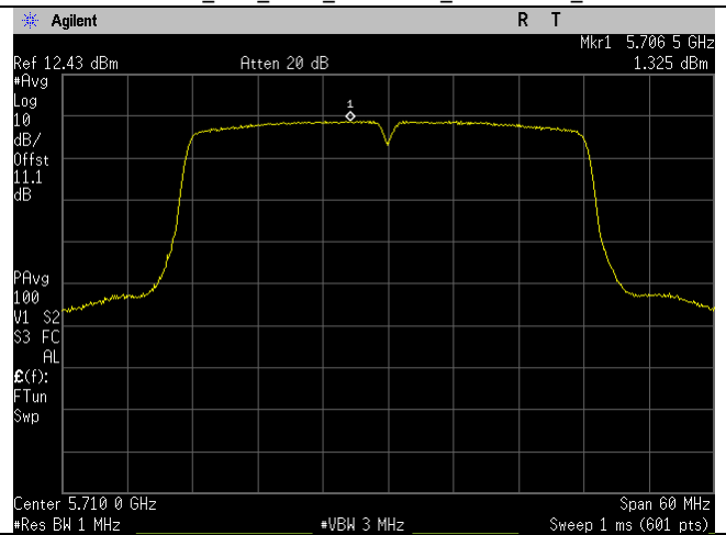
5710MHz_Ch_142_40MHz_n-mode Ant D
