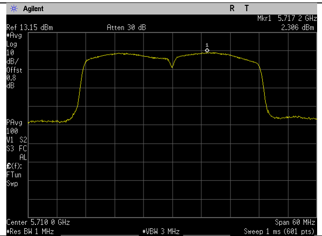
5710MHz_Ch_142_40MHz_n-mode_Ant B
