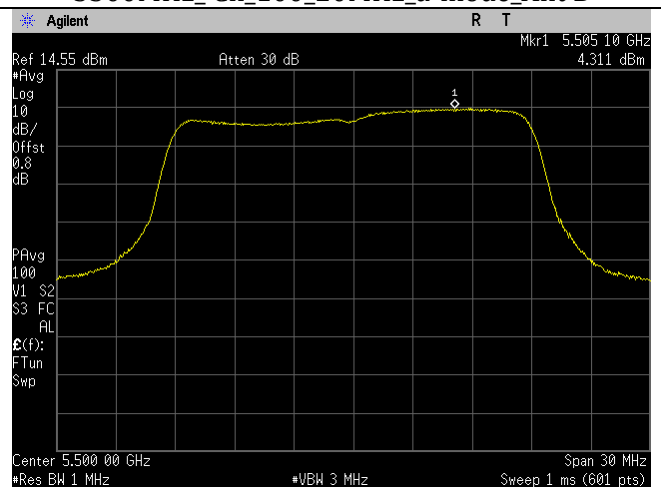
5500MHz_Ch_100_20MHz_n-mode_Ant B
