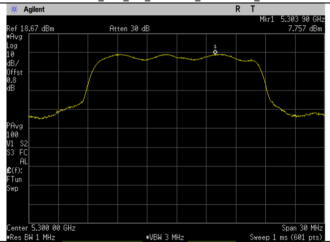
5300MHz_Ch_60_20MHz_a-mode_Ant B
