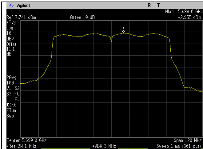
5690MHz_Ch_138_80MHz_ac-mode Ant C
