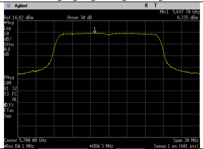
5700MHz_Ch_140_20MHz_a-mode_Ant B
