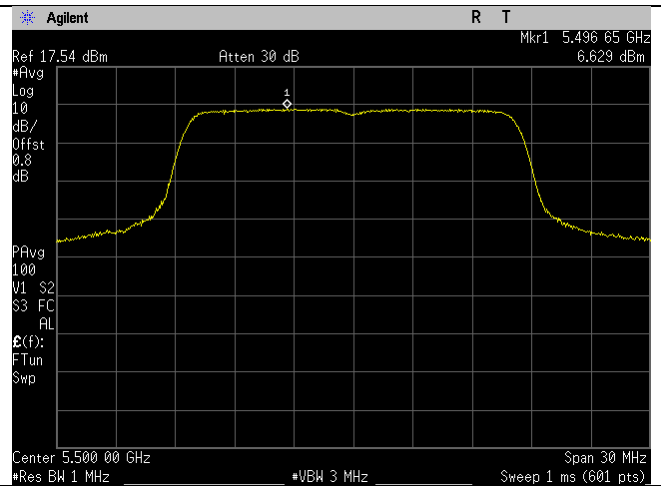
5500MHz_Ch_100_20MHz_a-mode_Ant B
