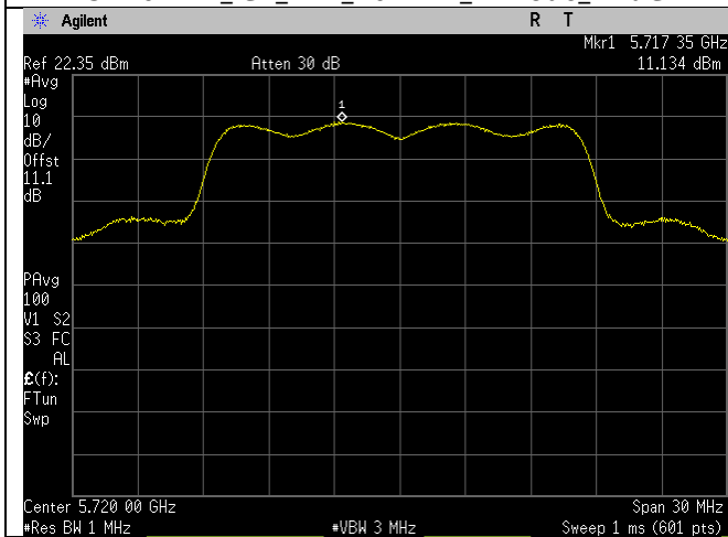
5720MHz_Ch_144_20MHz_a-mode Ant C
