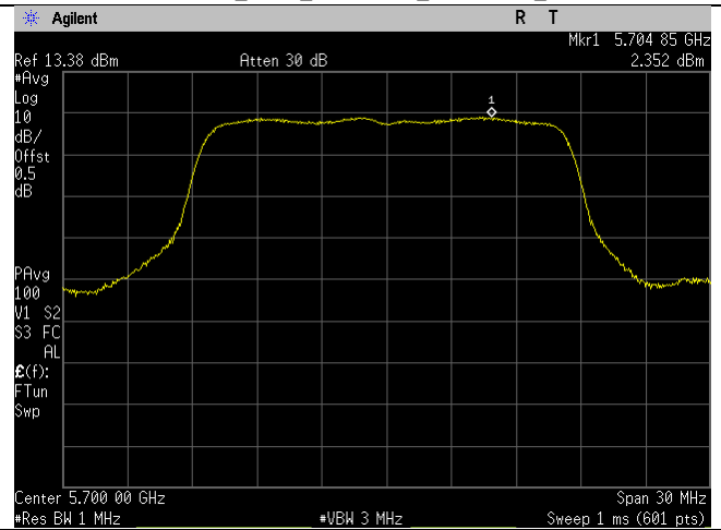
5700MHz_140_20MHz_a-mode_Ant D
