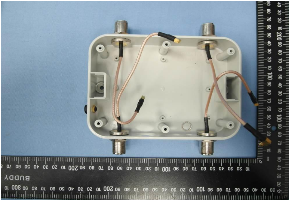
EUT Photo (19)
