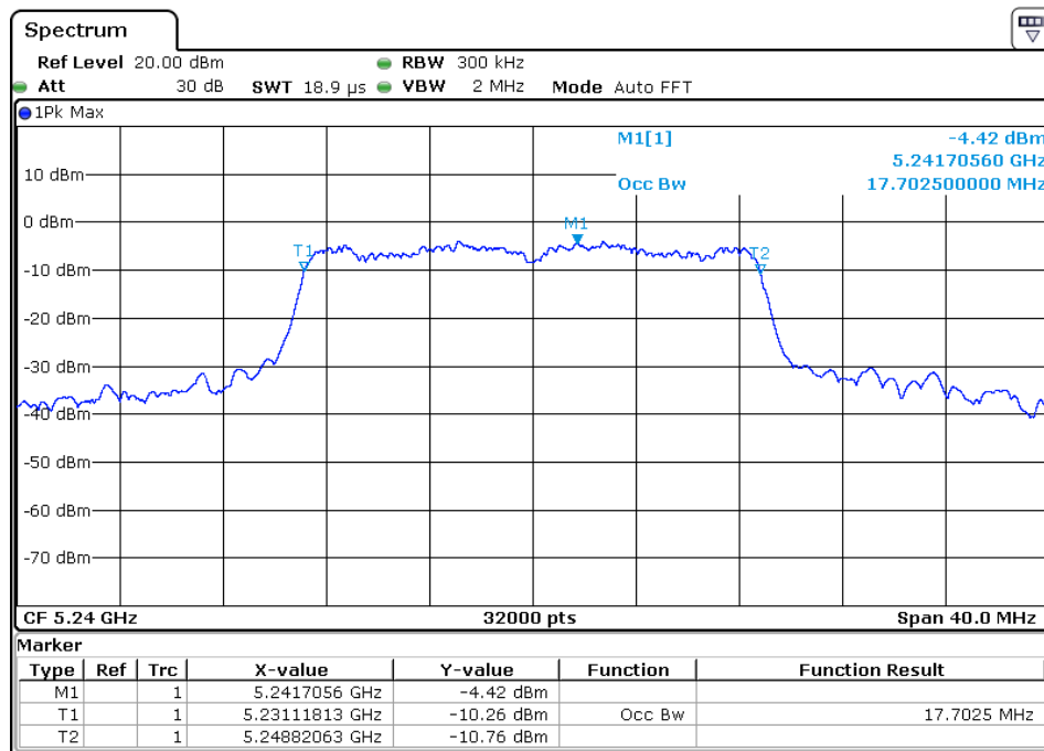
Ant 1 802.11 n20
