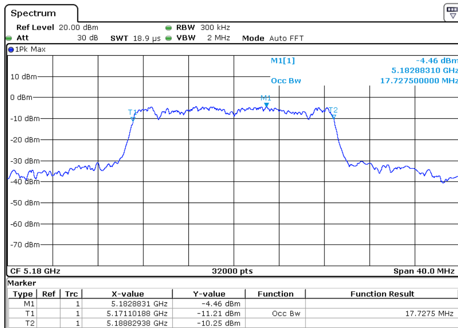
Ant 1 802.11 n20
