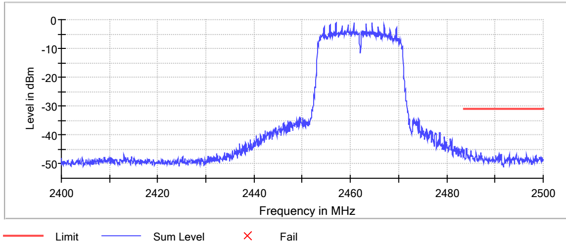
Band Edge
