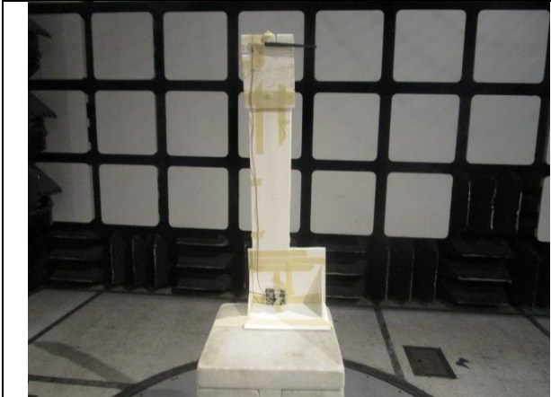
X EUT Orientation
