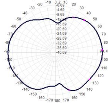
900.0MHz Total(E1-XZ), Max=-0.90dBi
