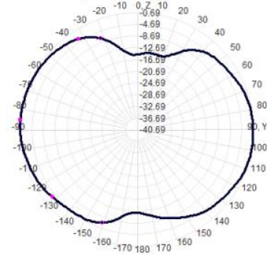
900.0MHz Total(E2-YZ), Max=-0.69dBi
