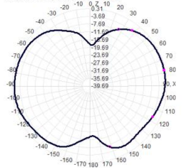
915.0MHz Total(E1-XZ), Max=-0.61dBi
