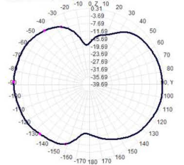
915.0MHz Total(E2-YZ), Max=0.16dBi
