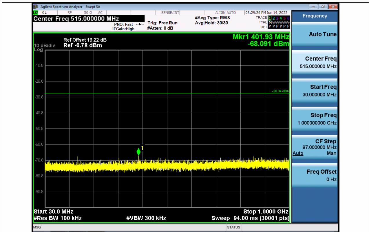
11G-Ant1-2462-30~1000-PASS
